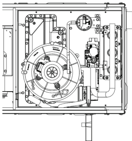
FIGURE 18 - ÉVACUATION HORIZONTALE À DROITE ET OPTION DE DRAINAGE CONTINU
