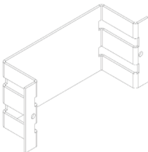
FIGURE 3 - SUPPORT POUR LE PURGEUR INTERNE
