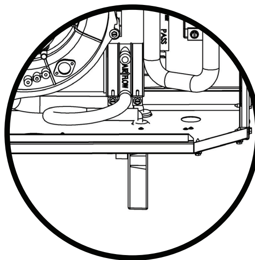
FIGURE 18 - ÉVACUATION HORIZONTALE À DROITE ET OPTION DE DRAINAGE CONTINU
