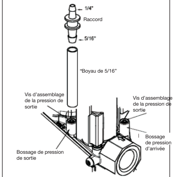
FIGURE 29 - ENSEMBLE DE VÉRIFICATION DE LA PRESSION DE LA SOUPAPE
