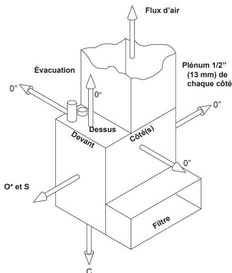
TABEAU B - DÉGAGEMENTS MINIMAUX AUX MATÉRIaux COMBUSTIBLES
