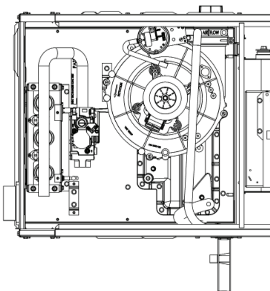
FIGURE 17 - ÉVACUATION HORIZONTALE À GAUCHE ET OPTION DE DRAINAGE
