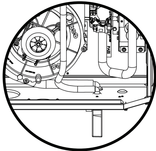
FIGURE 18 - ÉVACUATION HORIZONTALE À DROITE ET OPTION DE DRAINAGE
