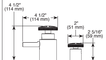
HW7532▲ Wheel Handles
