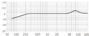
频率响应: (0dB=1V/Pa, 1KHz)
