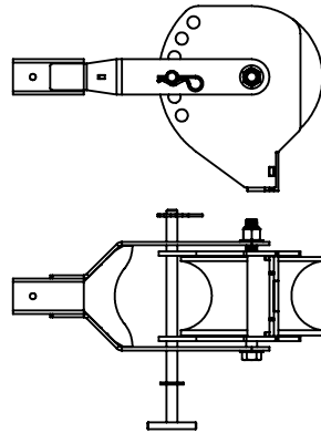
MODEL: CGS-40 STOCK: 59893201
