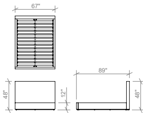
QUEEN BED EL-E006-Q
