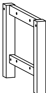
LEG (L&R Same) QTY 2
