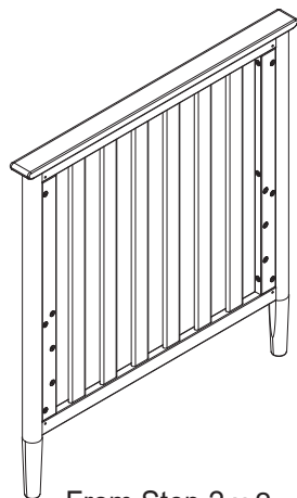
From Step 2 x 2 À partir de l'étape 2 x 2 Desde el paso 2 x 2
