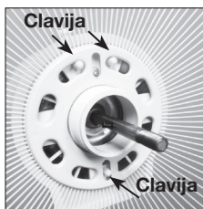
Arme la parrilla trasera en la caja del motor. La parrilla trasera debe entrar en las clavijas en la caja del motor como se muestra en la foto.
