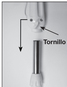
Ponga el ensamblado del motor/panel de control en el extensor de cromo y ajuste la tuerca manual.
