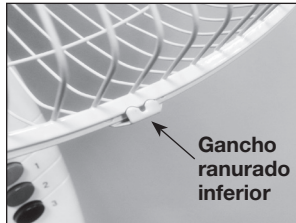
Con el logotipo hacia arriba, conecte la rejilla delantera a la rejilla trasera. Comience por insertar La rejilla delantera en el gancho ranurado inferior.
