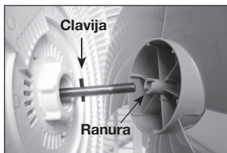
Quite cualquier cubierta protectora en el eje antes de instalar la hoja del abanico. Ponga la hoja del abanico en el eje del motor. Ver que la clavija del eje del motor debe entrar en las ranuras de la hoja del abanico.
