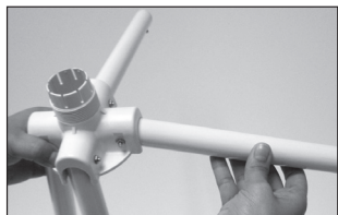
Endereza las patas de la base Quad-Pod®
