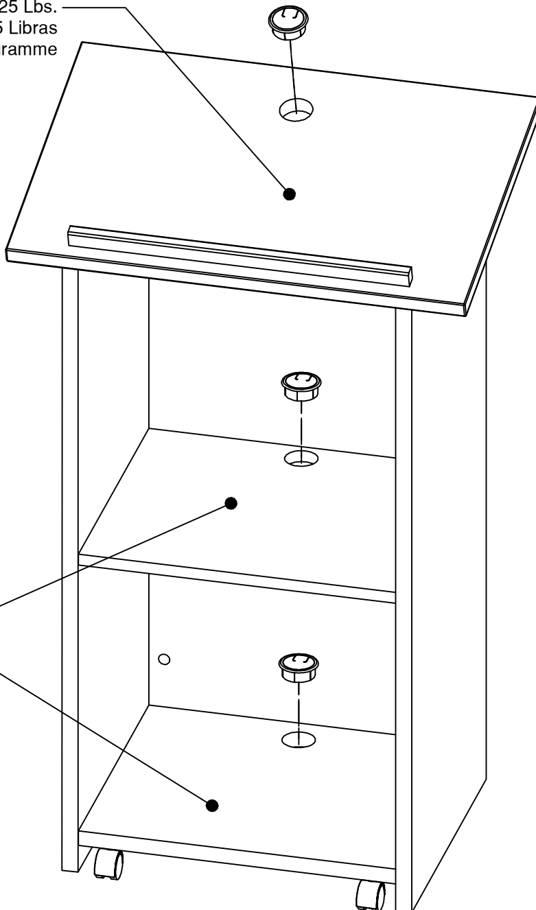
Grommet
