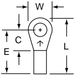
M18-6R/S Stud Size: 6 Wire Range: 22-18
