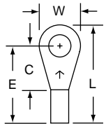
M18-8R/L Stud Size: 8 Wire Range: 22-18
