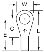
M18-10R/L Stud Size: 10 Wire Range: 22-18
