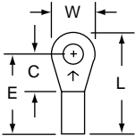
M18-4R/S Stud Size: 4 Wire Range: 22-18
