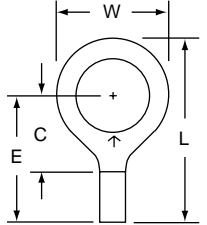
M18-38R Stud Size: 3/8 Wire Range: 22-18
