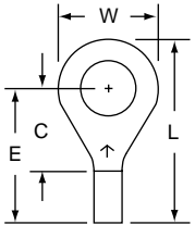
M18-14R/S Stud Size: 1/4 Wire Range: 22-18
