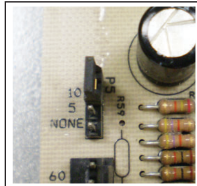
FIGURE 38 - FIL DE DÉRIVATION P5
