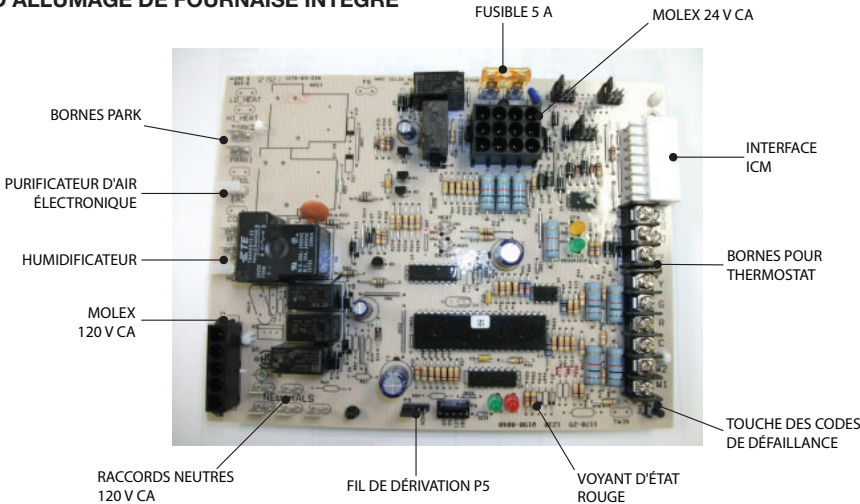
FIGURE 36 - CONTRÔLE D'ALLUMAGE DE FOURNAISE INTÉGRÉ
