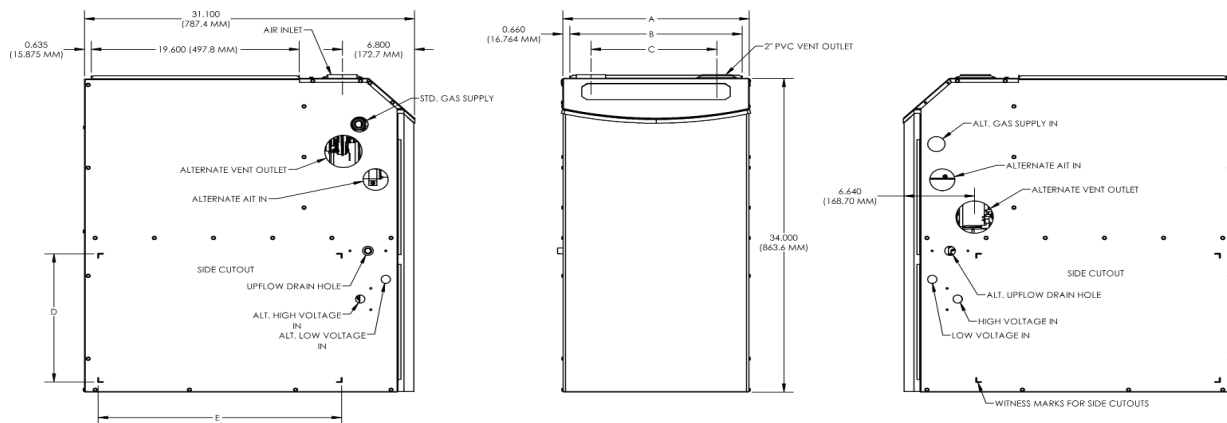
TABEAU A - DIMENSIONS DE LA FOURNAISE
