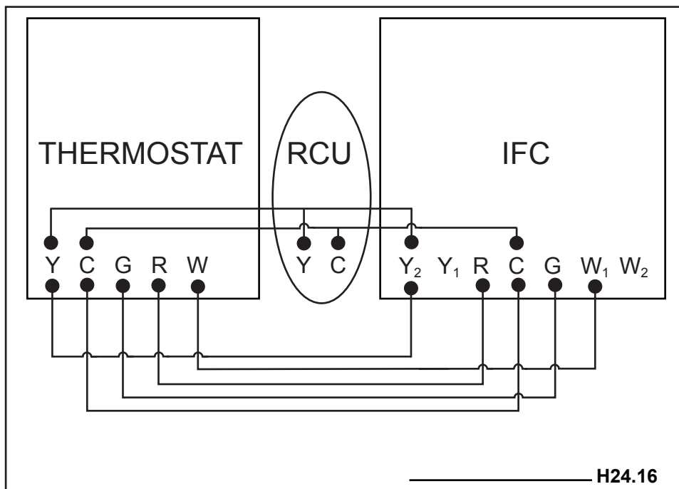
FIGURE 30 - DIAGRAMME DU CONNECTION DU THERMOSTAT
