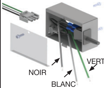
FIGURE 35 - BRANCHEMENTS ÉLECTRIQUES/CONNECTEUR MOLEX
