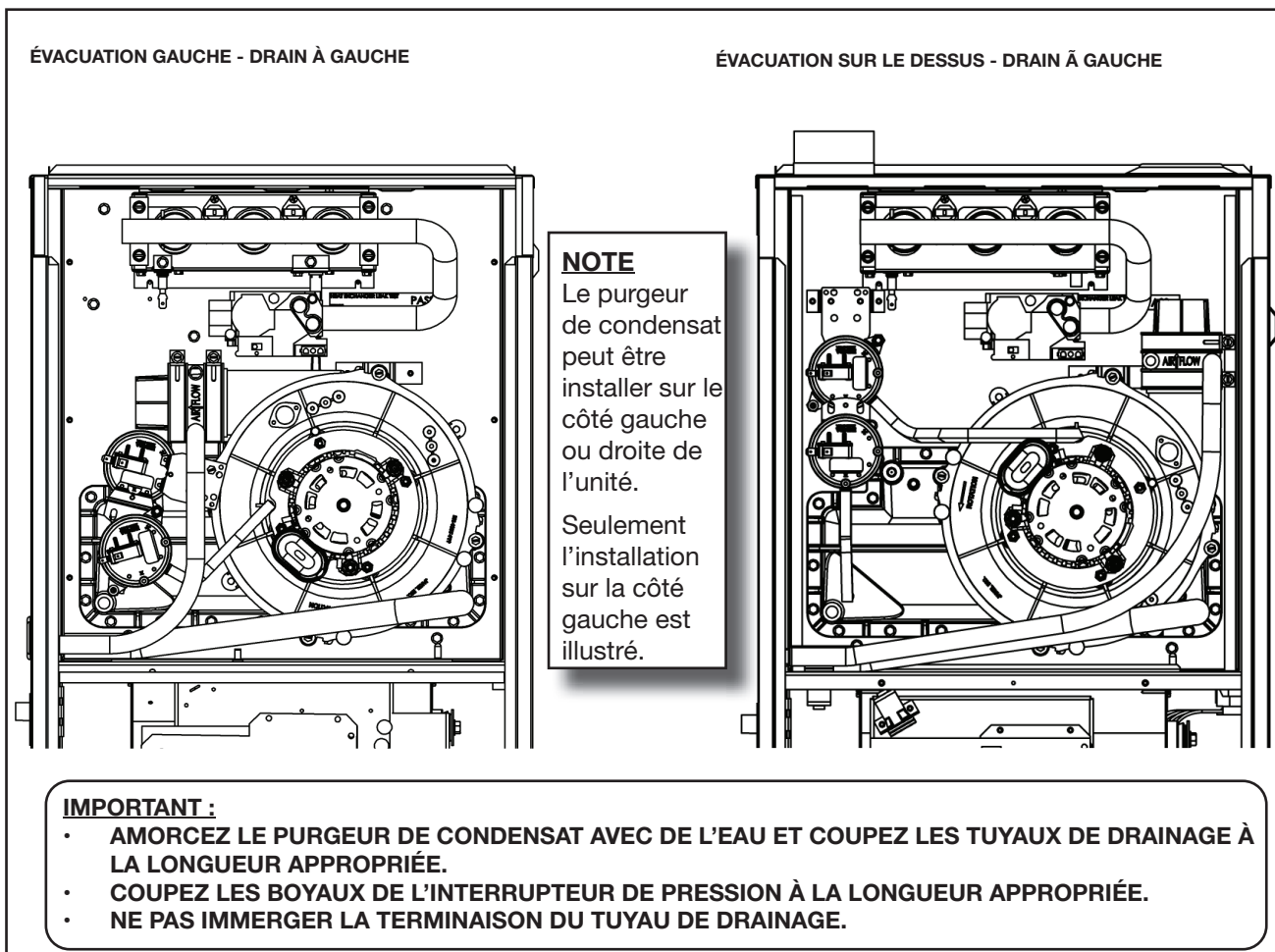
FIGURE 16 - OPTION D'ÉVACUATION ASCENDANTE ET DE DRAINAGE
