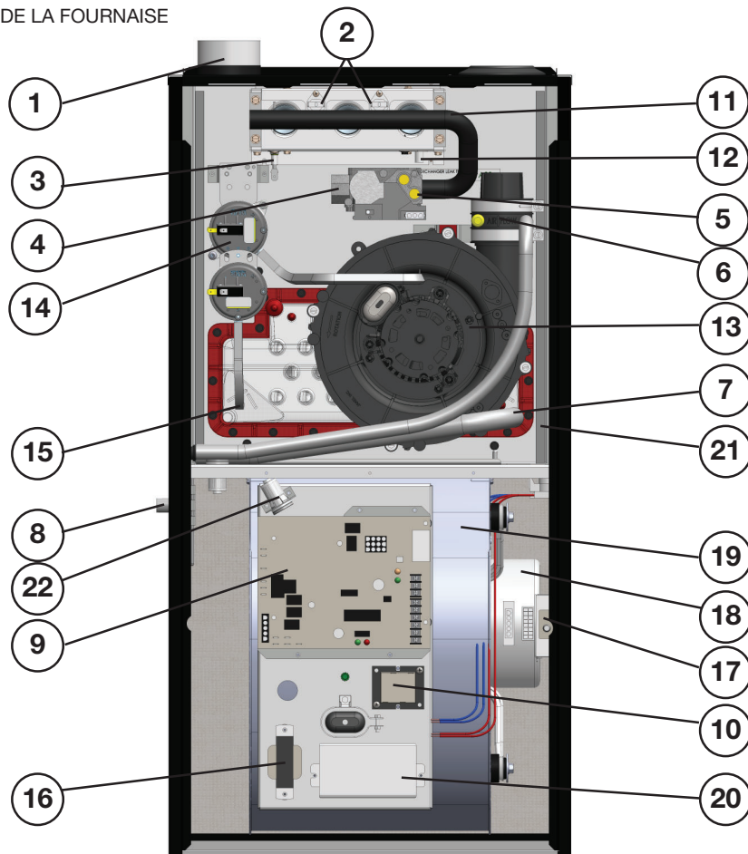
FIGURE 1 - COMPOSANTS DE LA FOURNAISE
