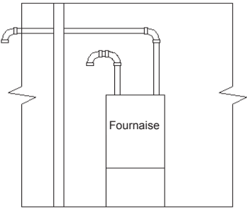
FIGURE 7 - PRISE D'AIR COMBURANT INDIRECTE
