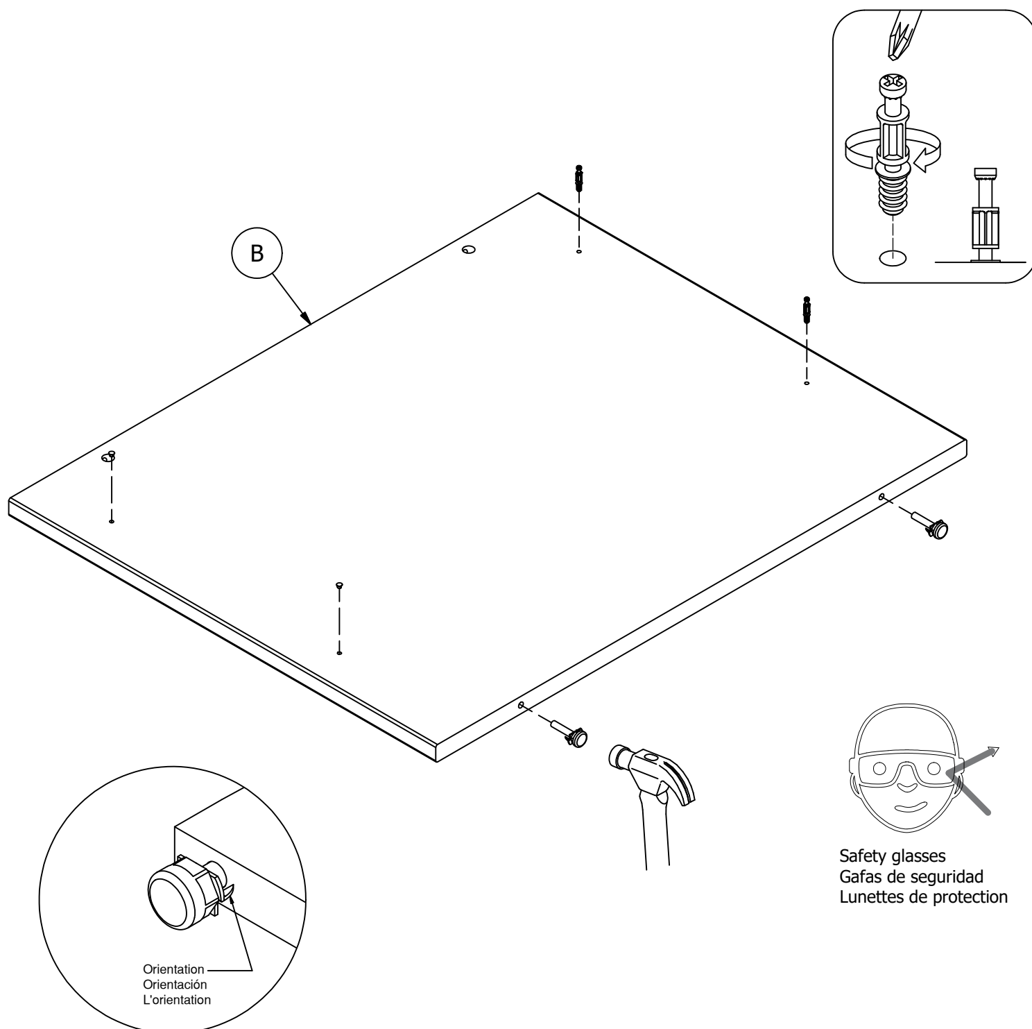
Leveler
