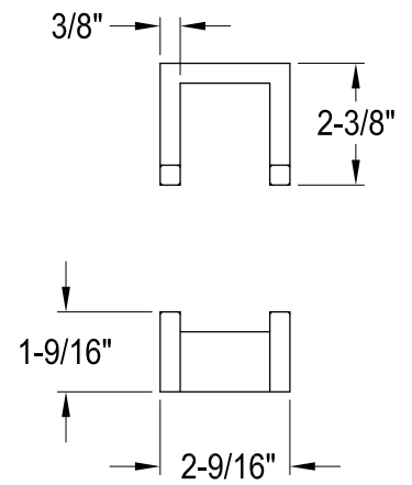
Robe Hook
