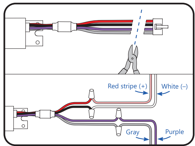
(D) Connect DC output using wire nuts.
