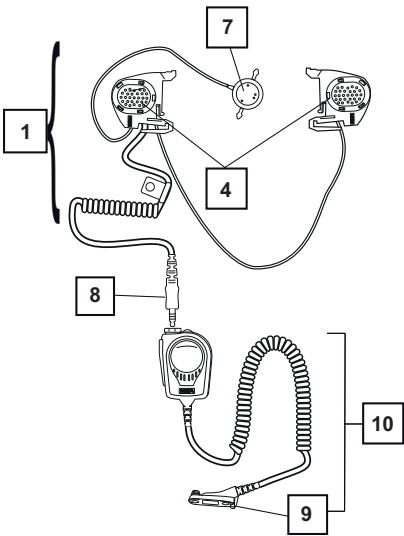
Figura 2 Osteofones, com condução do som pelos tecidos ósseos
