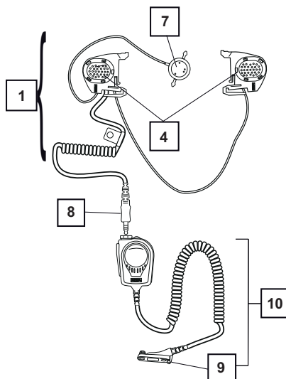
Figura 2 Sistema de comunicación de transmisión ósea
