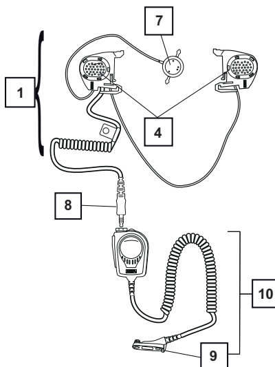
Obrázek 2 Komunikační systém s kostním vedením
