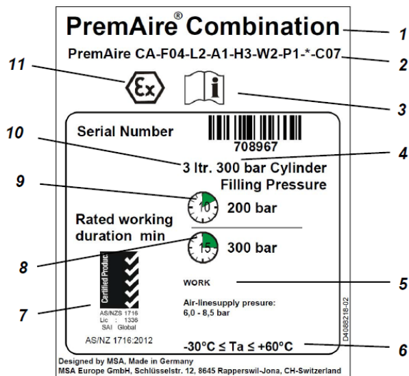
Abbildung 4 Gerätekarte PremAire Combination Mini nach AS/NZS 1716:2012
