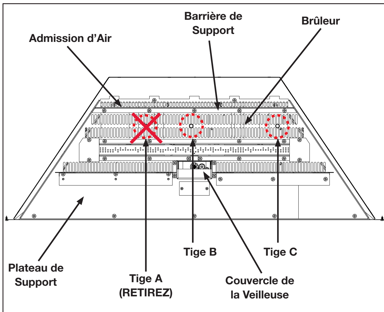
Vue d'Ensemble de Brûleur
