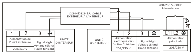
Schéma de connexion (9 K/12 K/18 K/24 K)
