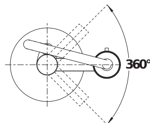
Swivel range
