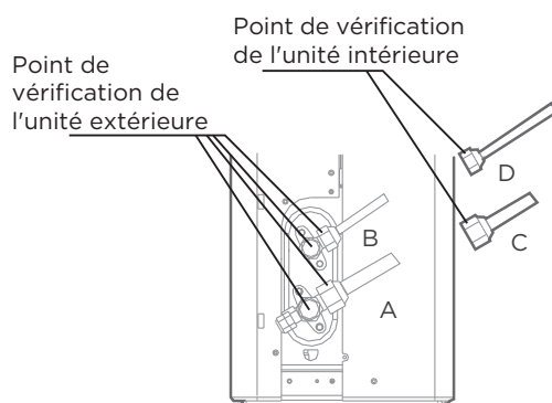
A : Vanne d'arrêt basse pression B : Vanne d'arrêt haute pression C ET D : Écrous évasés de l'unité intérieure
