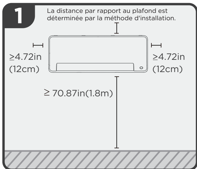
Sélectionner l'emplacement de l'installation
