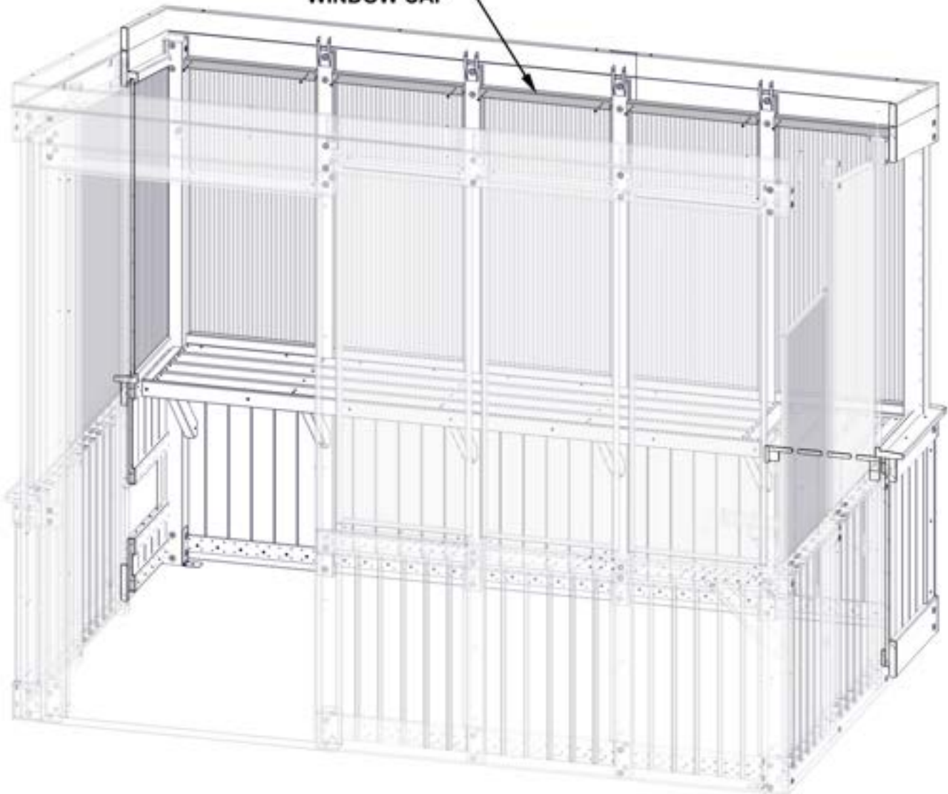
P02 (x5) WINDOW CAP
