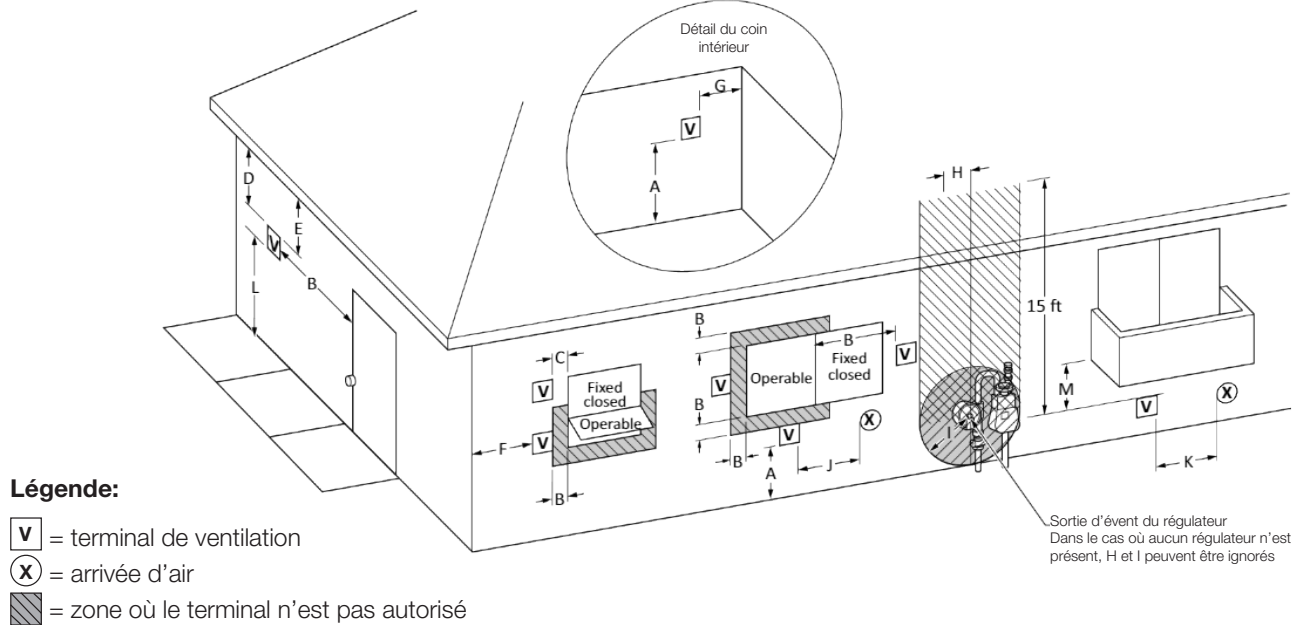
FIG. 4.2.1 - DÉGAGEMENT DE LA TERMINAISON DU SYSTÈME D'ÉVENT DIRECT
