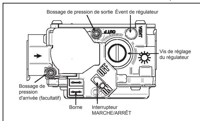
FIG. 28. - SOUPAPE DE GAZ WHITE RODGERS 36J24-214 (W010-2614)
