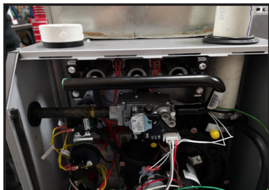
FIGURE 24 - ENSEMBLE DE BRÛLEUR À ALLUMAGE SIMULTANÉ
