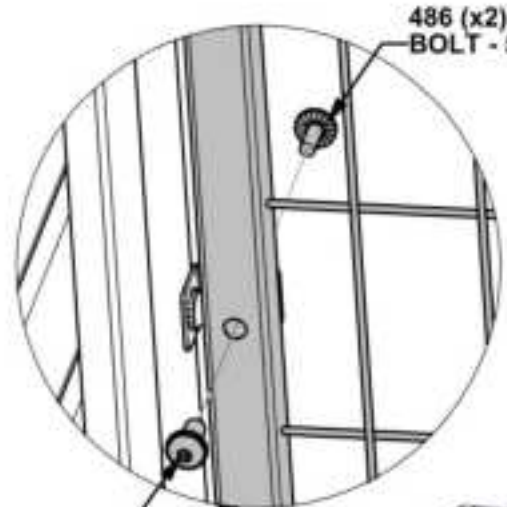
404 (x2) BARREL NUT - 5/8"
