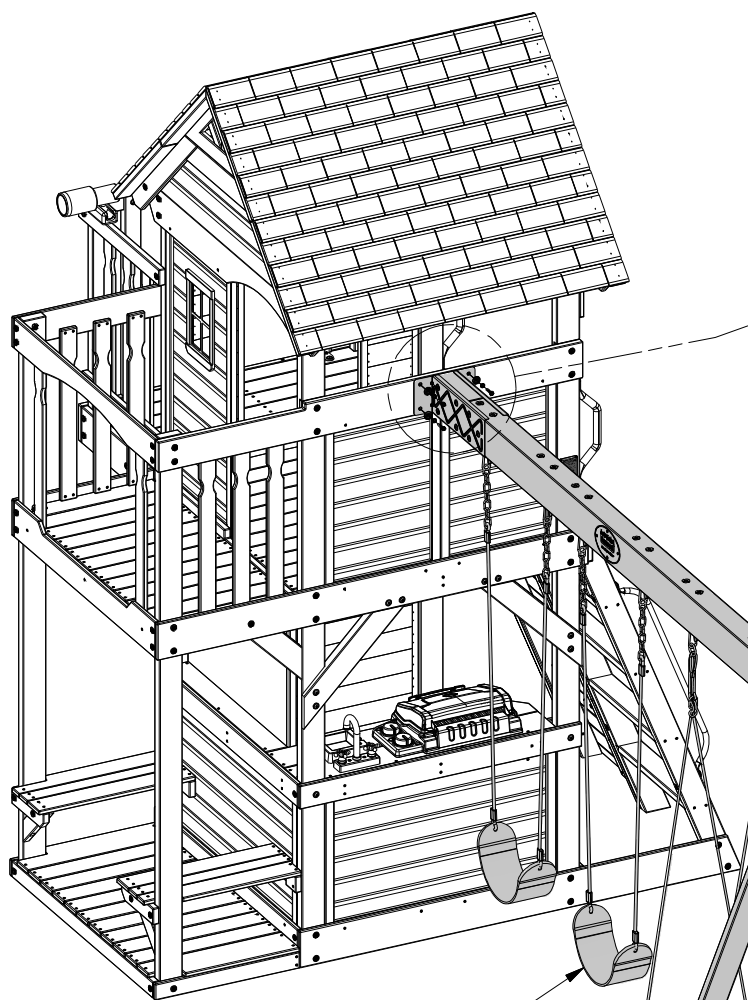
397 (x2) SWING
