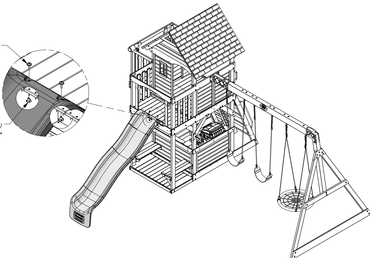
468 (x2) BOLT - 1"
