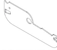
L03 LOUVER SIDE PLATE - A4M02334 (x39) 1/16"x2 3/16"x6 9/16" (2x55x167)
