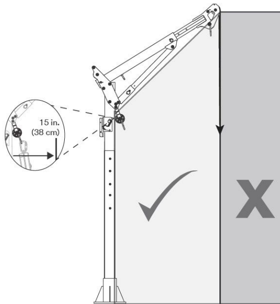
Rysunek 5 — Bezpieczny obszar roboczy
