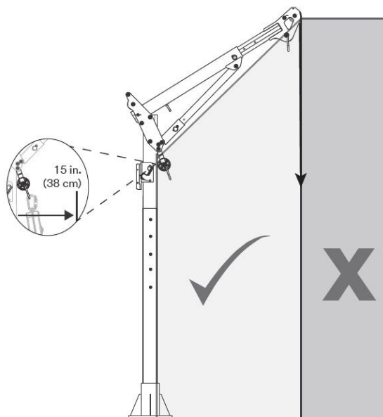
Figura 5 – Área de trabalho segura
