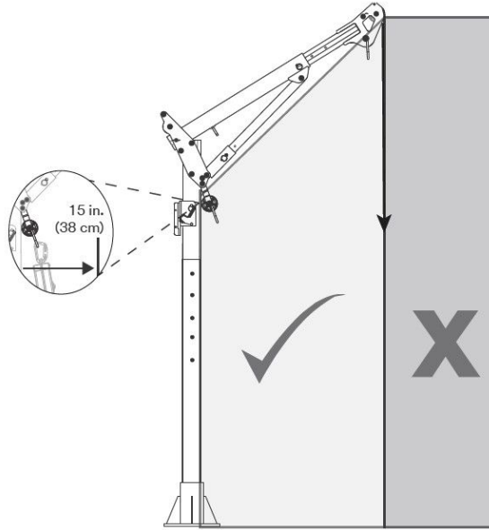
그림 5 - 안전 작업 영역
