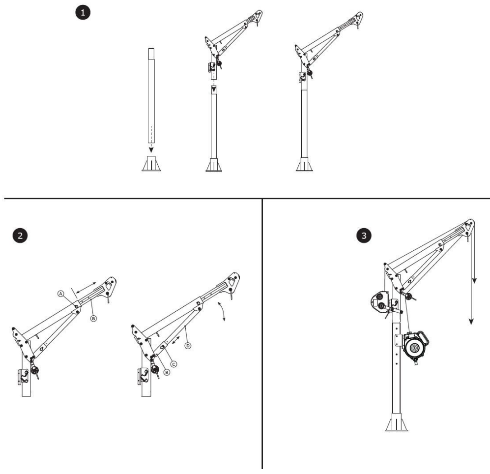
Figure 7 – Installation du système de potence
