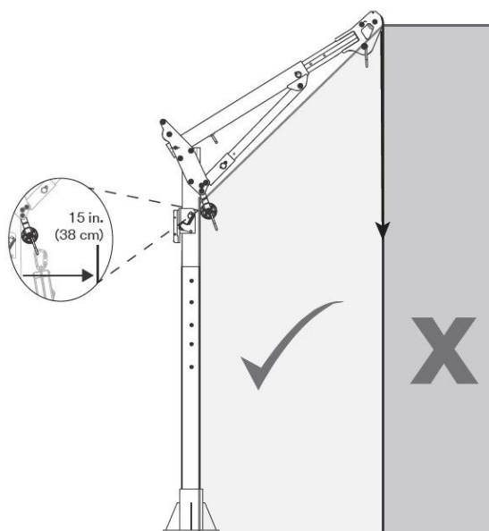
Obrázok č. 5 – Bezpečný pracovný priestor
