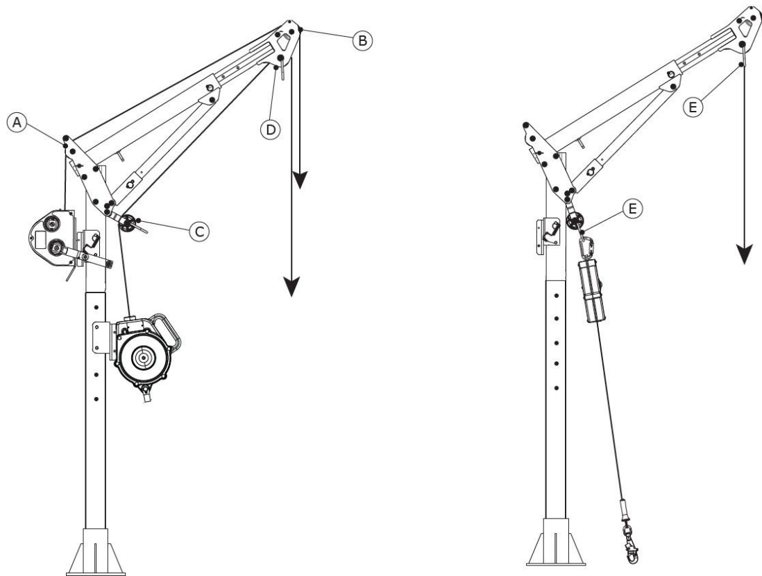
Figura 8: Fijación del sistema secundario de conexión
