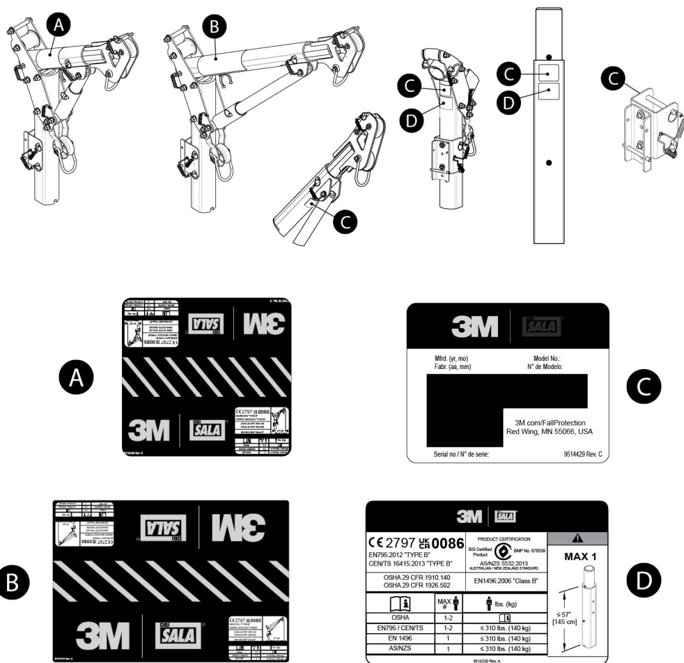
図10 - 製品ラベル
