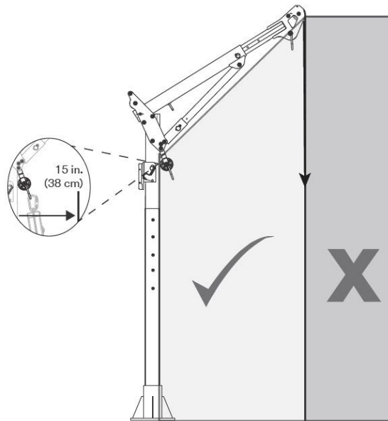
図5 - 安全作業区域
