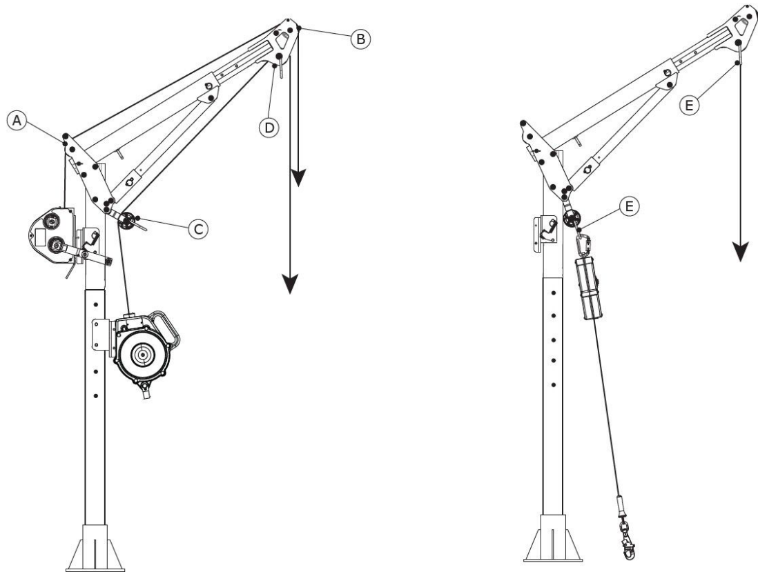
Figure 8 : Sécurisation du sous-système d'amarrage
