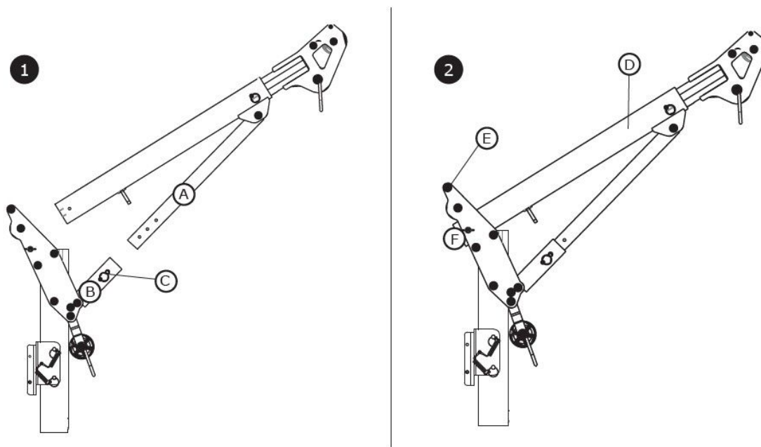
Figura 6 - Configurazione del gruppo
