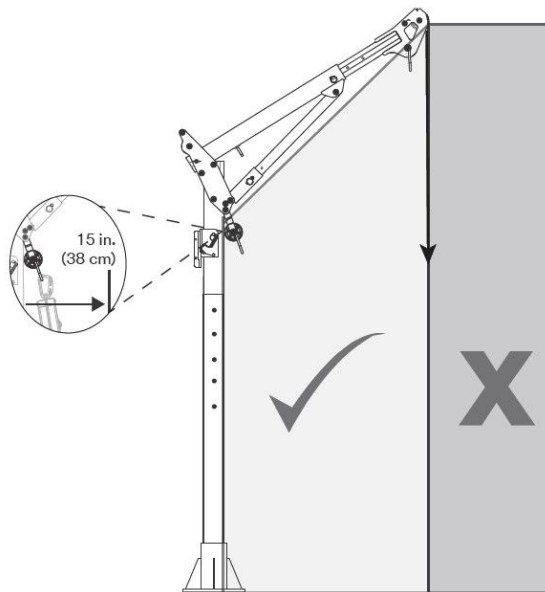
Figure 5 - Area di lavoro sicura
