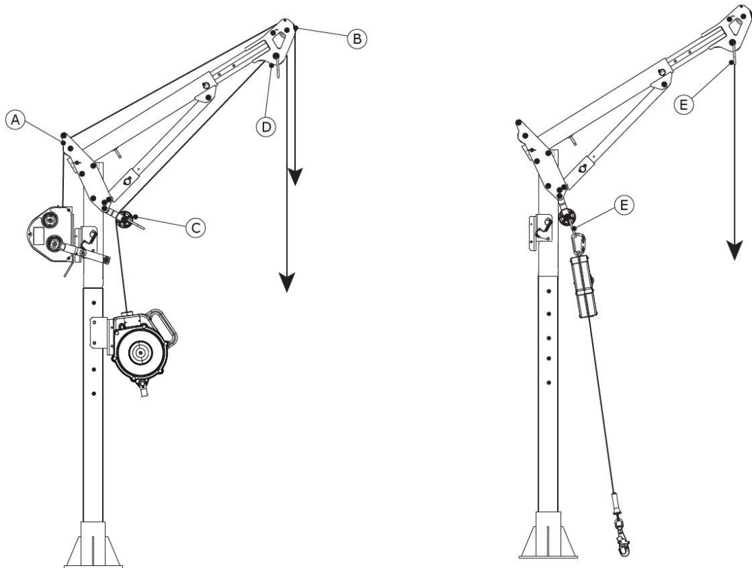
Εικόνα 8 - Ασφάλιση του συνδετικού υποσυστήματος
