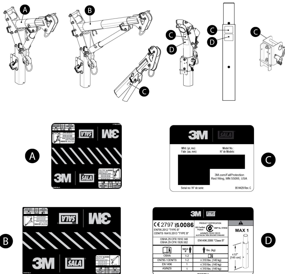
Abbildung 10 – Produktetiketten
