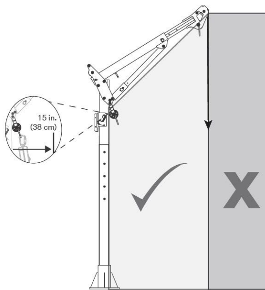
Figur 5 – Säkert arbetsområde
