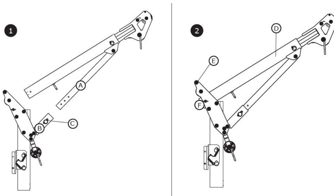
Obrázek 6 – Konfigurace sestavy
