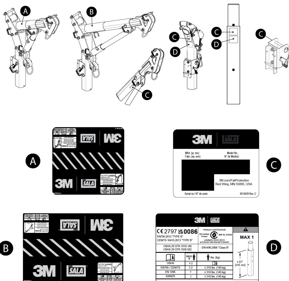
Mynd 10 – vörumerkingar
