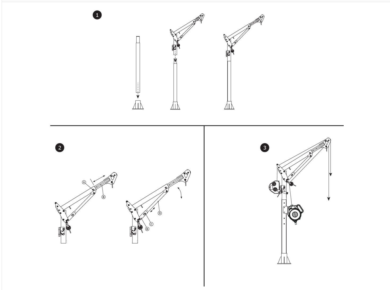
Figure 7 – Installation du système de bossoir
