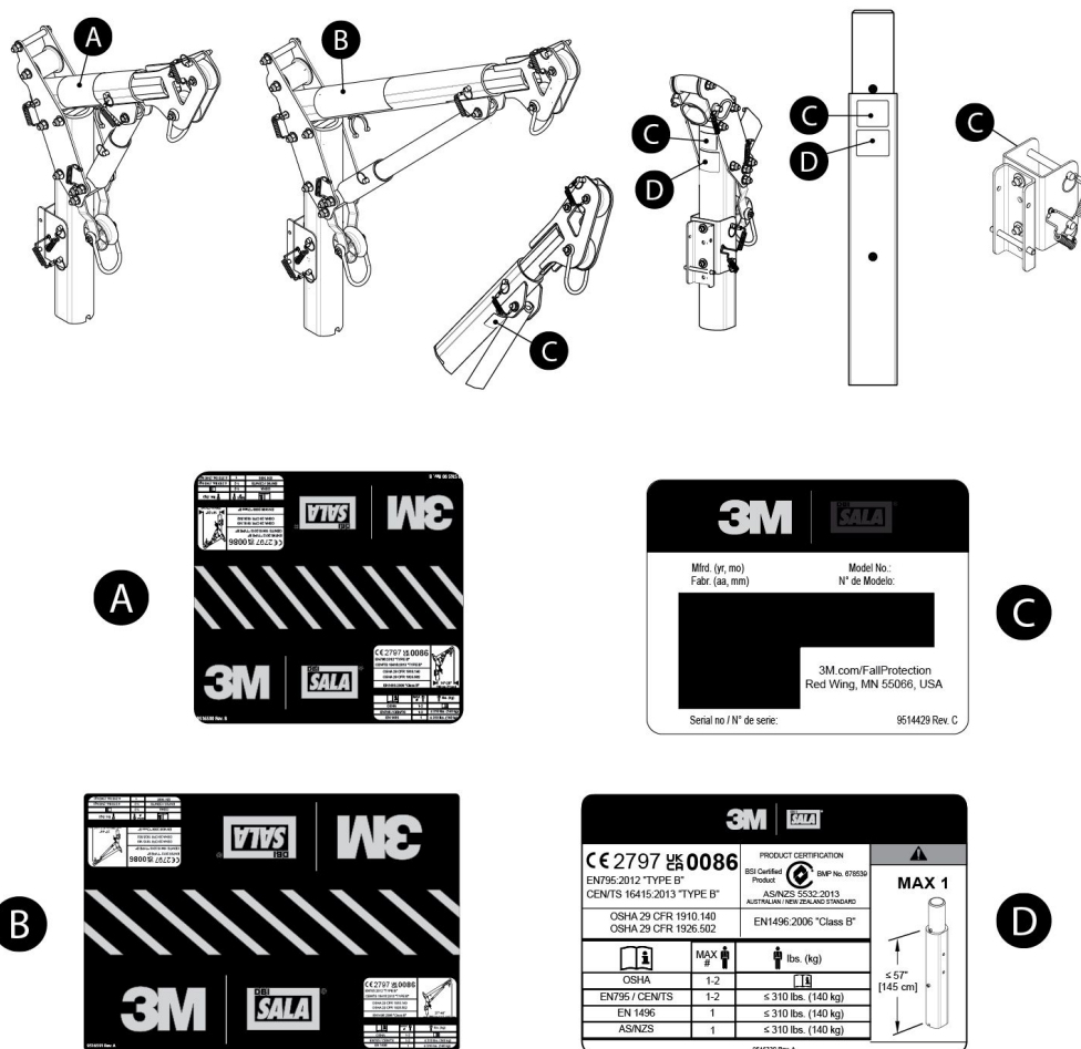
Afbeelding 10 - Productlabels
