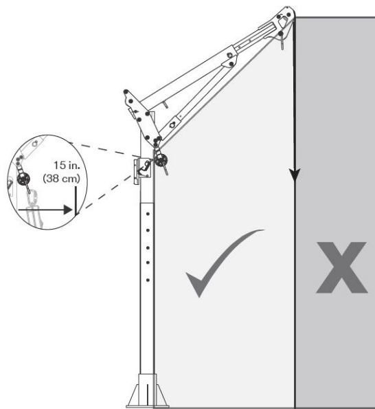
Joonis 5 - Ohutu tööpiirkond
