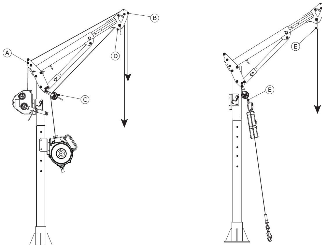
Slika 8. – Pričvršćivanje priključnog podsustava
