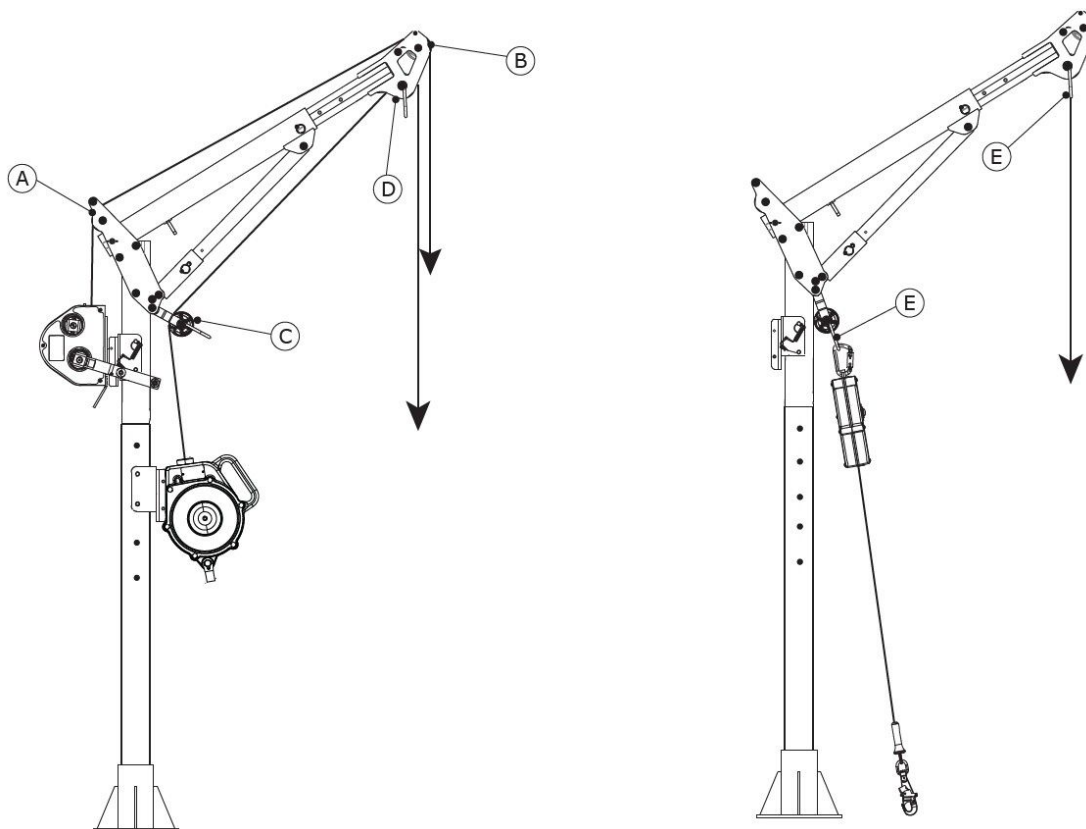
Figura 8 – Asigurarea subsistemului de conectare
