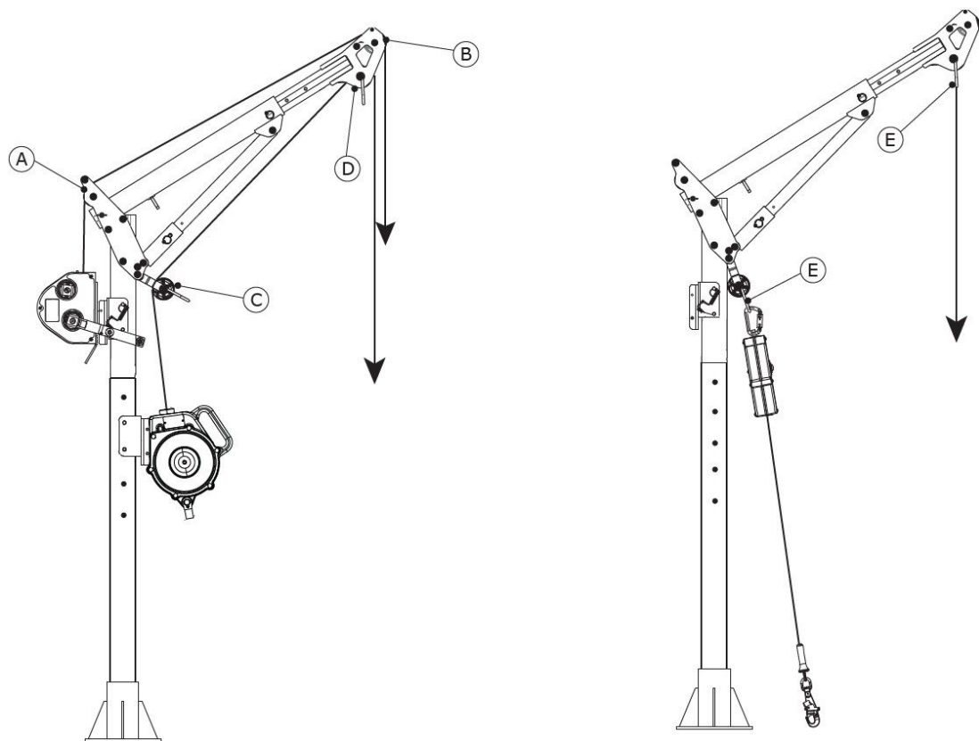
Фигура 8 – Закрепване на свързващата подсистема
