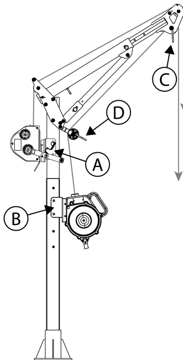
그림 9 - 마운팅 위치
