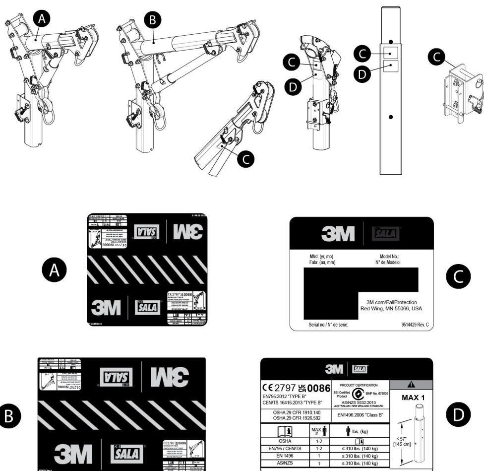
Figura 10 – Etichetele produsului
