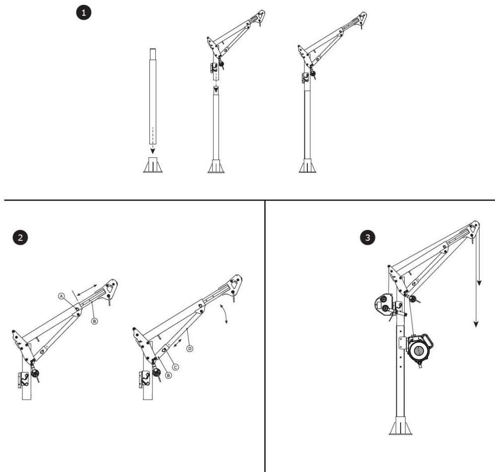
図7 - ダビットシステムの設置
