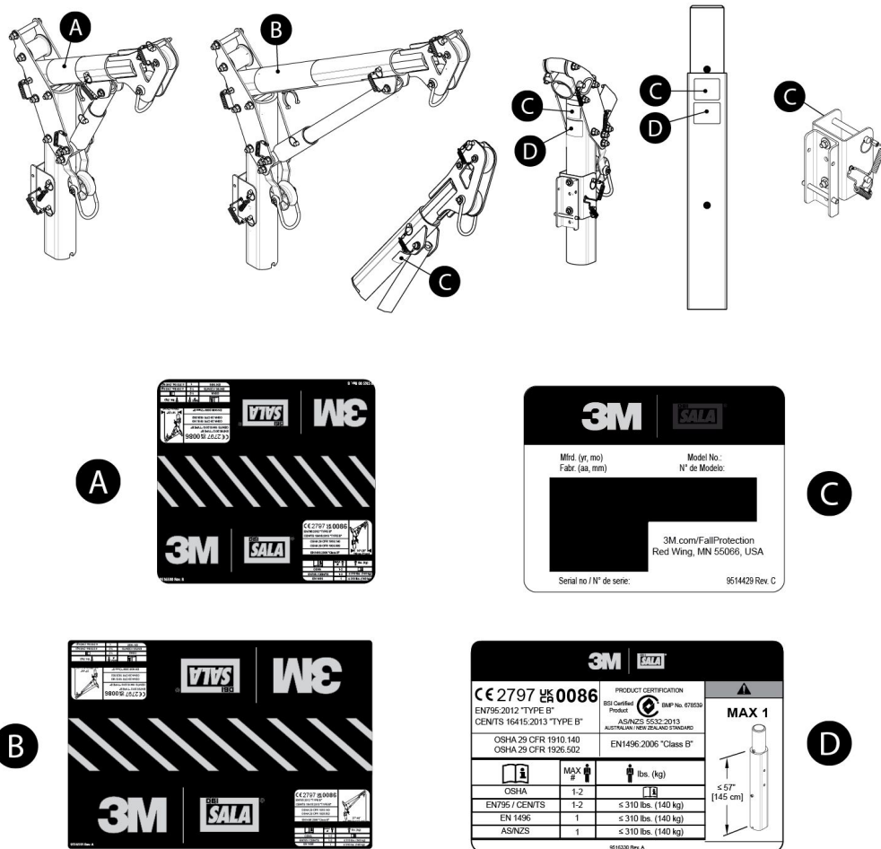
Kuva 10 – Tuotetarrat
