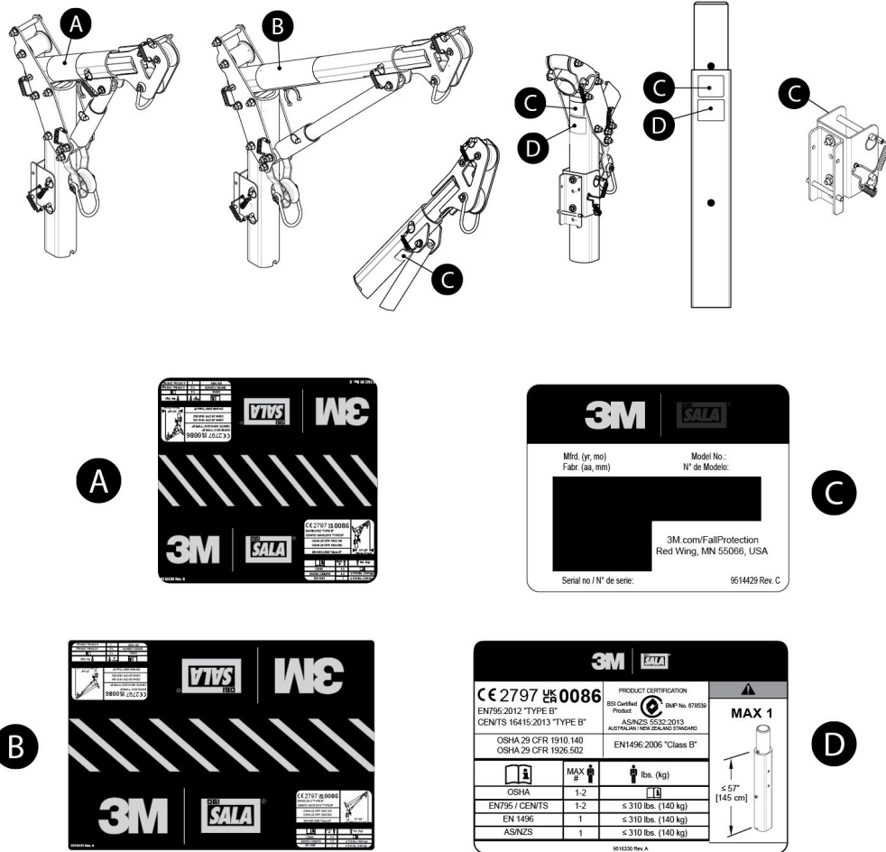
Şekil 10 - Ürün Etiketleri
