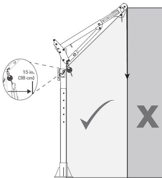
Figura 5: Área de trabajo segura
