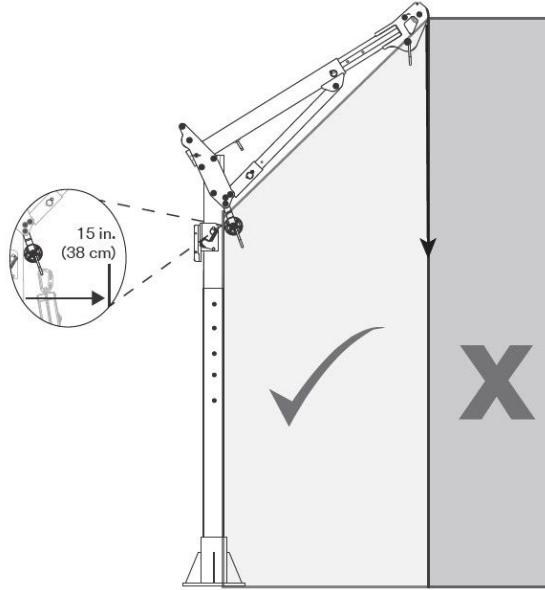
Şekil 5 - Güvenli Çalışma Alanı
