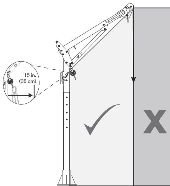
Figur 5 – Sikkert arbejdsområde
