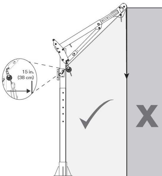
Фигура 5 – Безопасна работна зона
