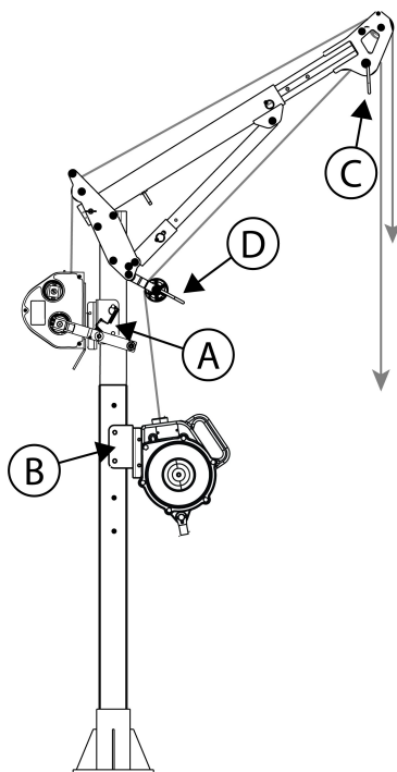
9. ábra - Rögzítési helyek
