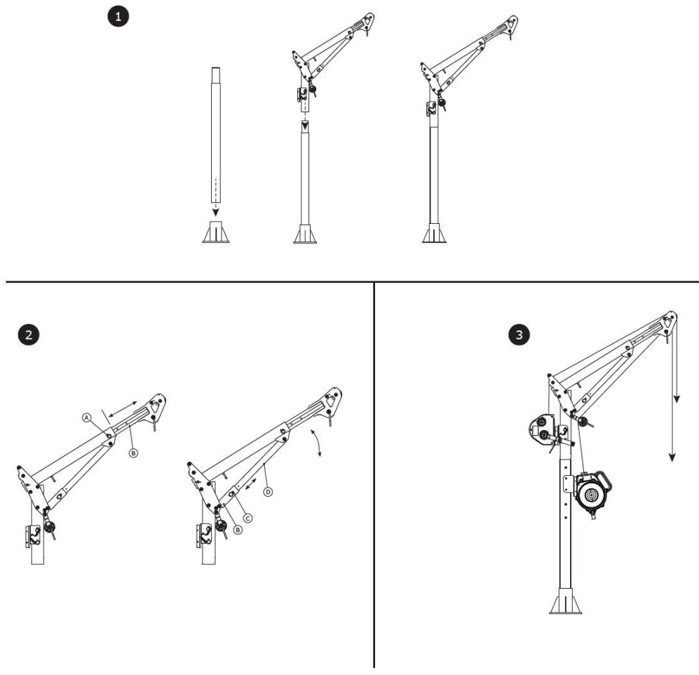
Figura 7 - Instalação do sistema Davit
