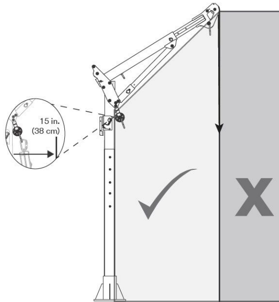
Kuva 5 – Turvallinen työalue
