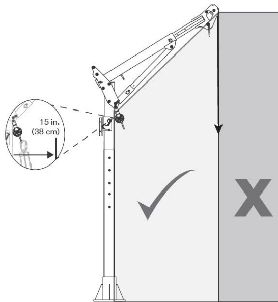
5. ábra – Biztonságos munkaterület
