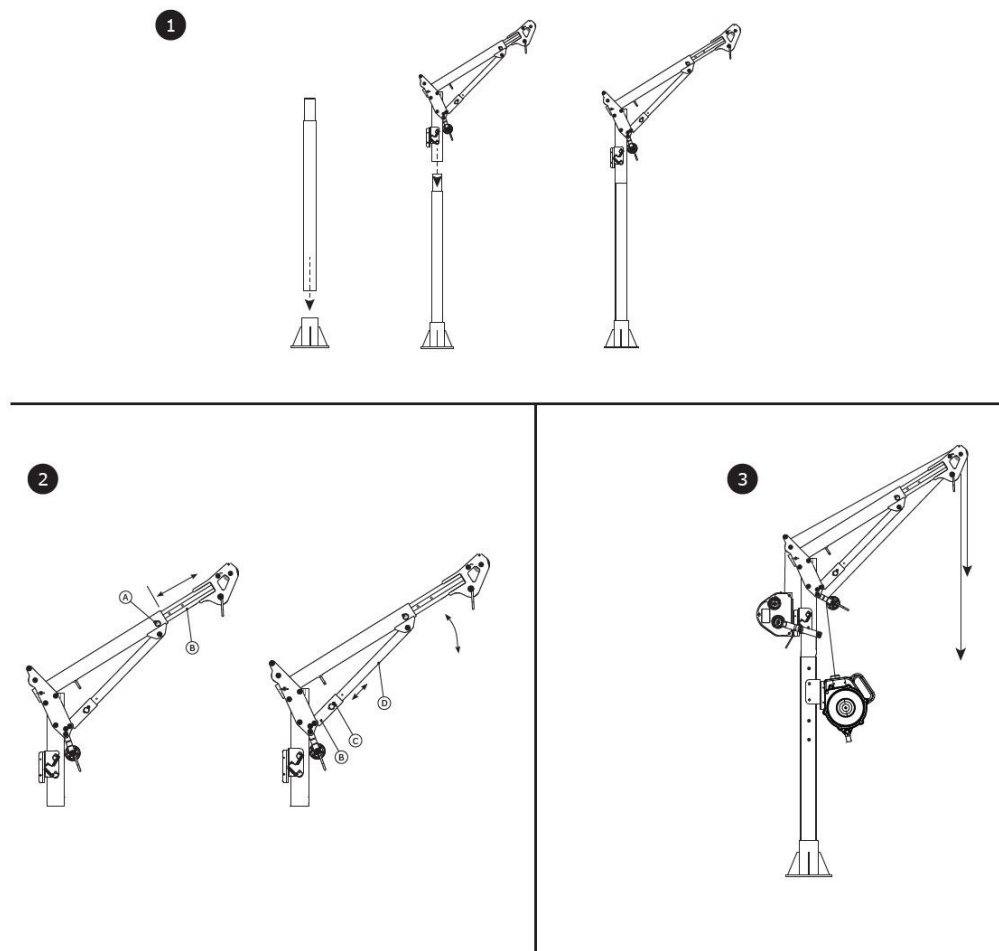
Фигура 7 – Монтаж на системата с кран тип Davit
