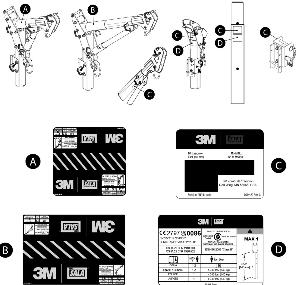
그림 10 - 제품 라벨
