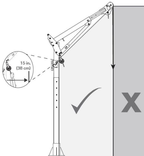
Afbeelding 5 - Veilig werkgebied
