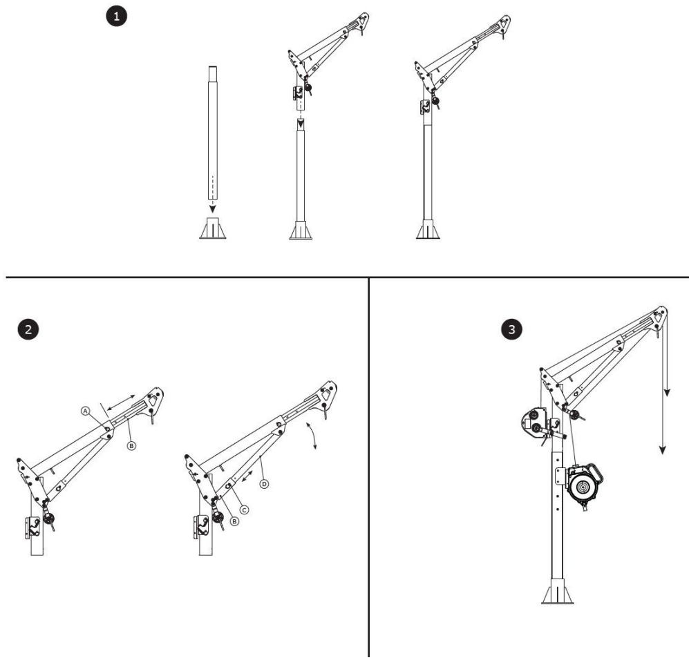
Figura 7: Instalación del sistema del pescante
