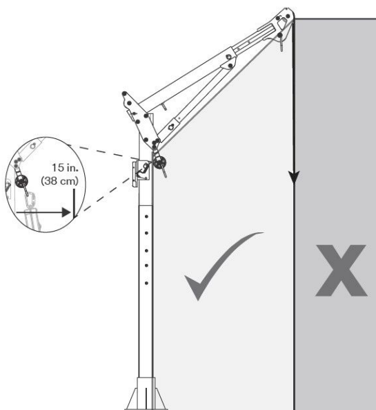
Mynd 5 – Öruggt vinnusvæði
