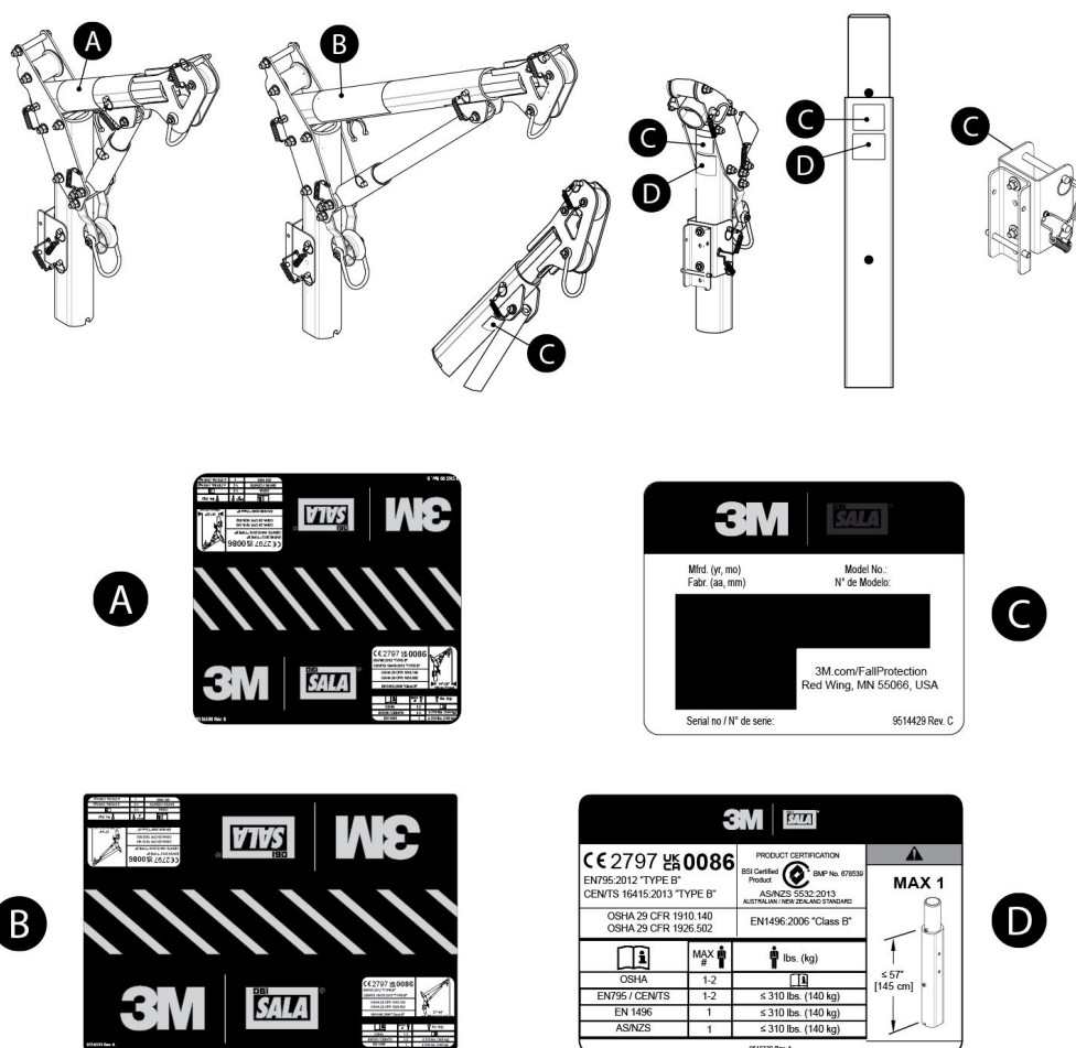
Figur 10 – Produktetiketter
