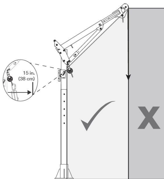
5. attēls — droša darba zona
