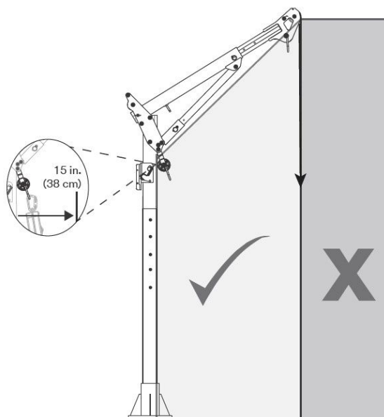
Slika 5 – Sigurno radno područje
