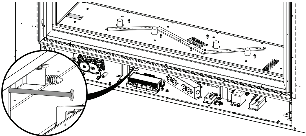
AIR SHUTTER ADJUSTMENT AJUSTEMENT DU VOLET D'AIR
