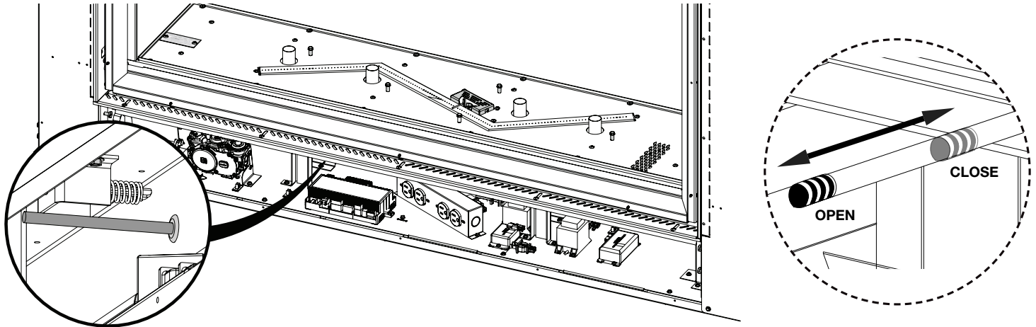
AIR SHUTTER ADJUSTMENT AJUSTEMENT DU VOILET D'AIR
