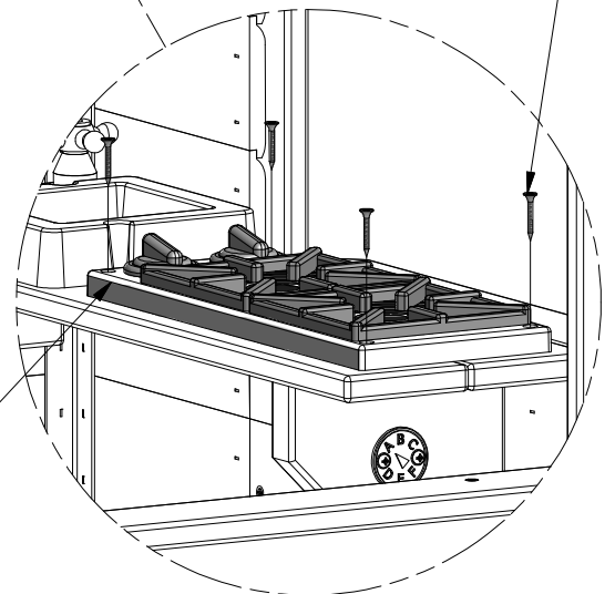
VITE PFH 8x1 1/8 (4 PLCS)
