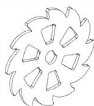
S02 SPROCKET - A4M02147 (x1) 3/16"x4 11/16"x4 11/16" (4x119x119)
