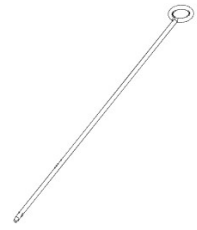
R03 HOLDING ROD - A4M02787 (x1) 1/4"x1 3/16"x21 7/16" (6x30x544)
