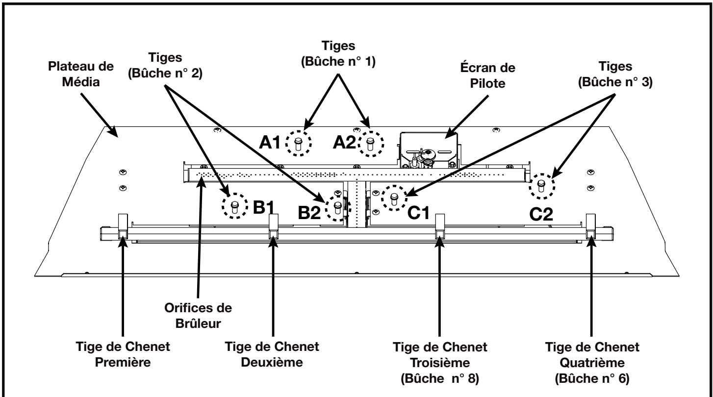
Vue d'Ensemble de Brûleur
