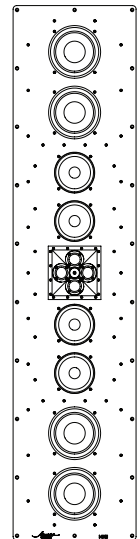
BE812 MKII
