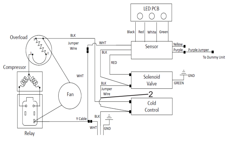
WIRING DIAGRAM - EZO 220V EI ESQUEMA que ALAMBRA - EZO 220V DIAGRAMME qui TELEGRAPHIE - EZO 220V
