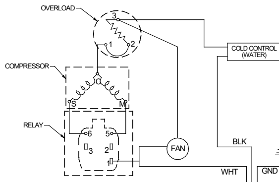
Fig. 15 115V Wiring Diagram
