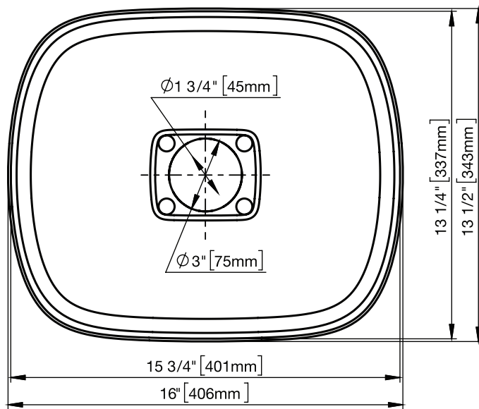
TOP VIEW / VISTA SUPERIOR / VUE DE HAUT
