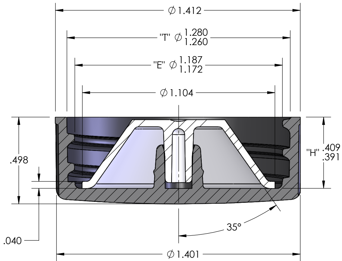
SECTION A-A
