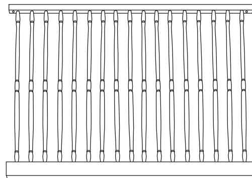
C. Crib Side (2) C. Côté du lit de bébé (2)
