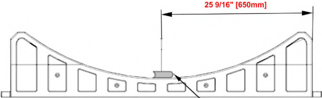
VUE AVANT
