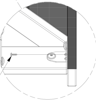
128 (x10) TORNILLO - 5/8
