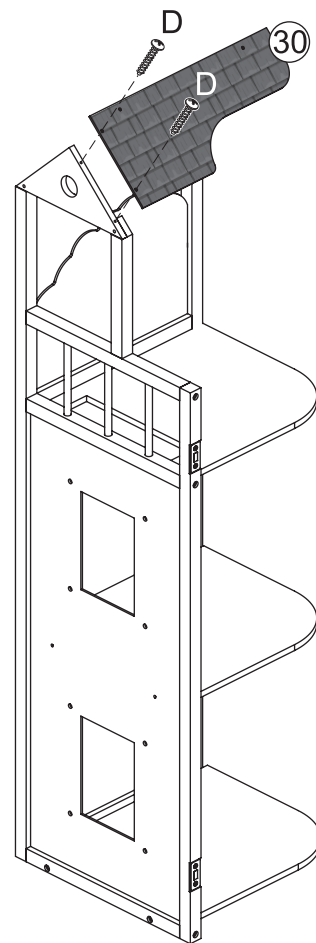
Back View / Vue Arrière / Vista Posterior / Rückansicht / vista posteriore
