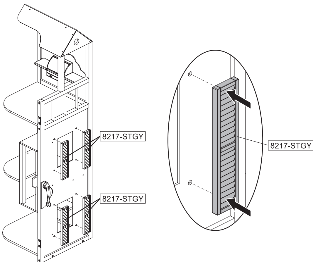
Outside View / Vue extérieure / Vista exterior / Außenansicht / Vista dall'esterno
