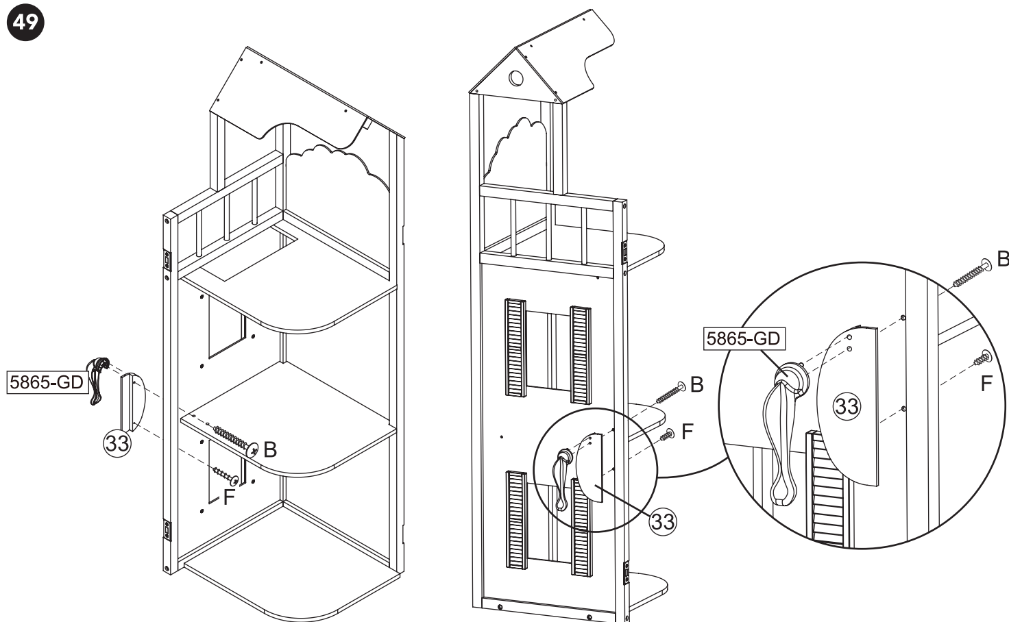
Outside View / Vue extérieure / Vista exterior / Außenansicht / Vista dall'esterno
