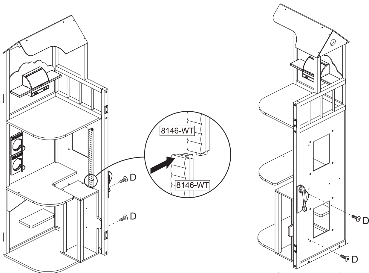
Outside View / Vue extérieure / Vista exterior / Außenansicht / Vista dall'esterno
