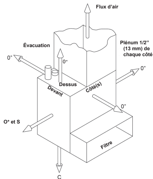
TABEAU B - DÉGAGEMENTS MINIMAUX AUX MATÉRIEAUX COMBUSTIBLES
