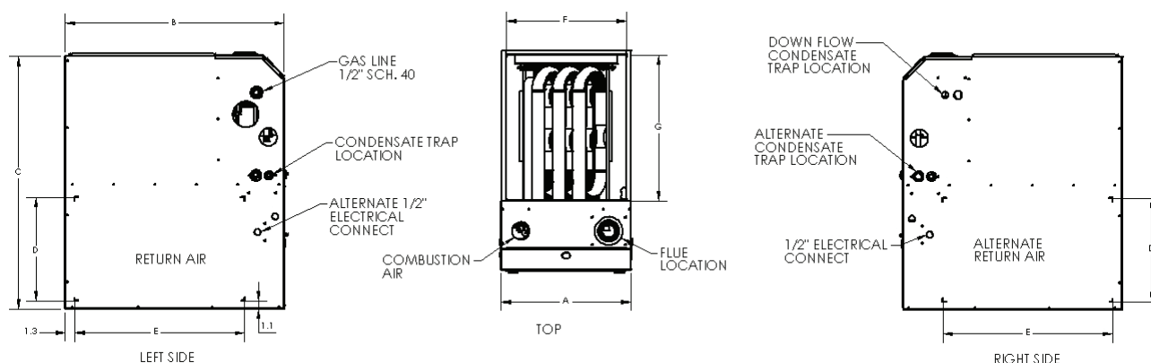
TABEAU A - DIMENSIONS DE LA FOURNAISE
