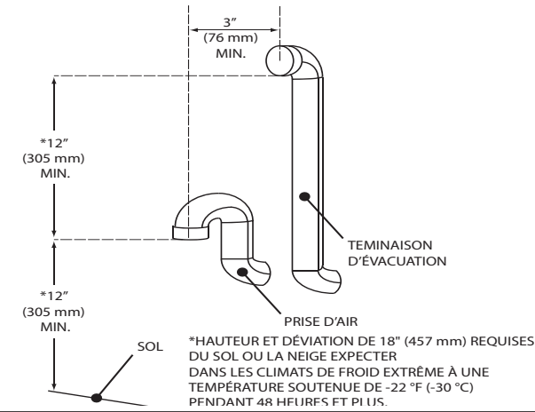
FIGURE 9 - DÉTAIL D'UN ÉVENT PÉRISCOPEIQUE
