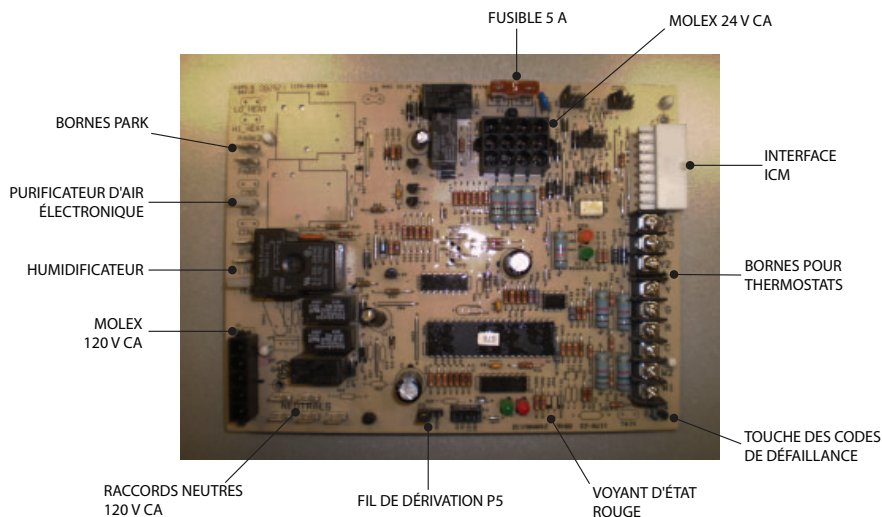
FIGURE 32A - CONTRÔLE D'ALLUMAGE DE FOURNAISE INTÉGRÉ
