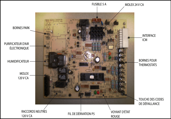
FIGURE 36 - CONTRÔLE D'ALLUMAGE DE FOURNAISE INTÉGRÉ
