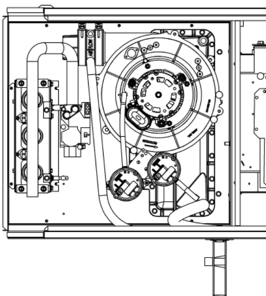
FIGURE 17 - ÉVACUATION HORIZONTALE À GAUCHE ET OPTION DE DRAINAGE CONTINU
