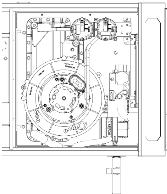
FIGURE 19 - ÉVACUATION DESCENDANTE ET DE DRAINAGE
