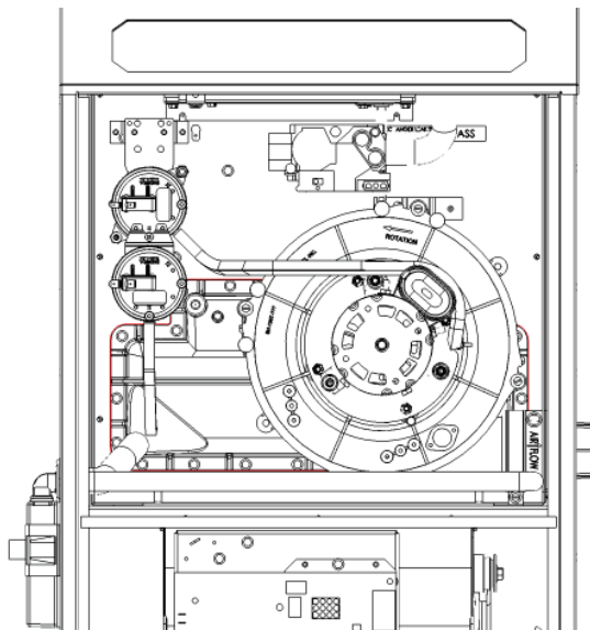
FIGURE 16 - OPTION D'ÉVACUATION ASCENDANTE ET DE DRAINAGE CONTINU
