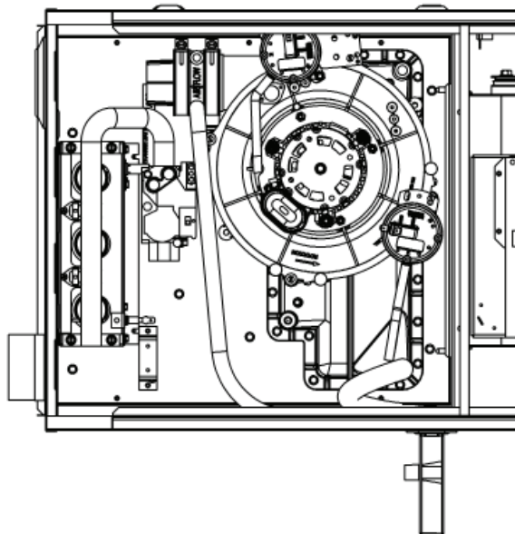
FIGURE 17 - ÉVACUATION HORIZONTALE À GAUCHE ET OPTION DE DRAINAGE INSTALLATION D'ÉVACUATION À DROITE (Panneau)
