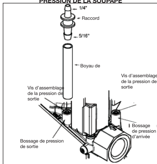
FIGURE 29 - ENSEMBLE DE VÉRIFICATION DE LA PRESSION DE LA SOUPE
