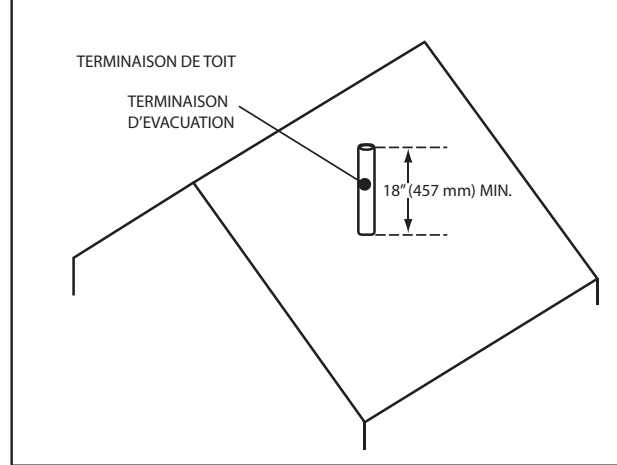
FIGURE 10 - ÉVACUATION VERTICALE
