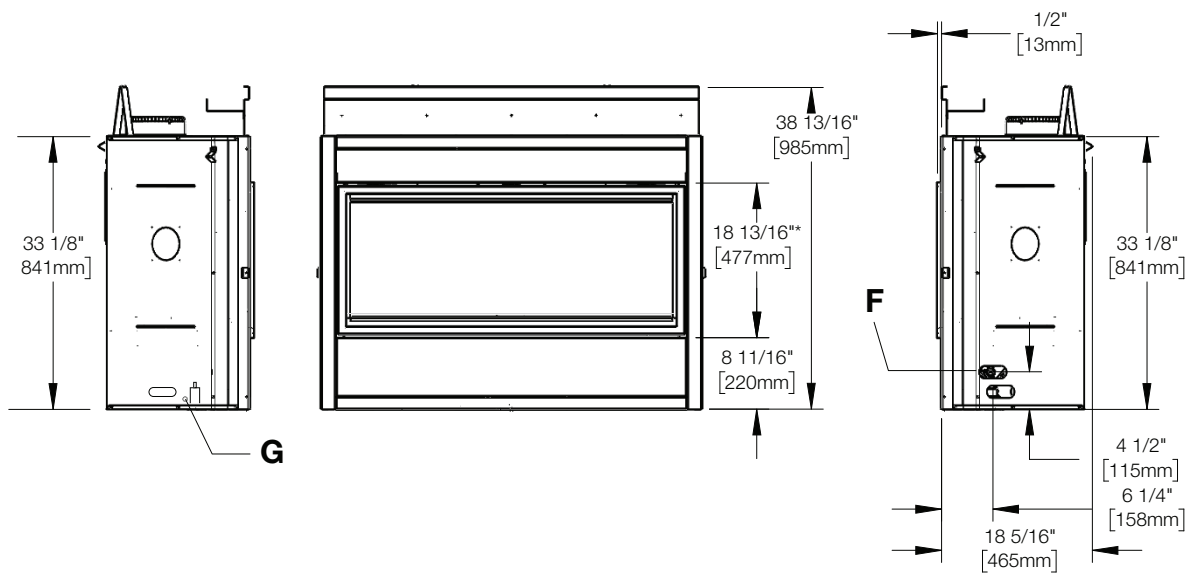
Vue avant
