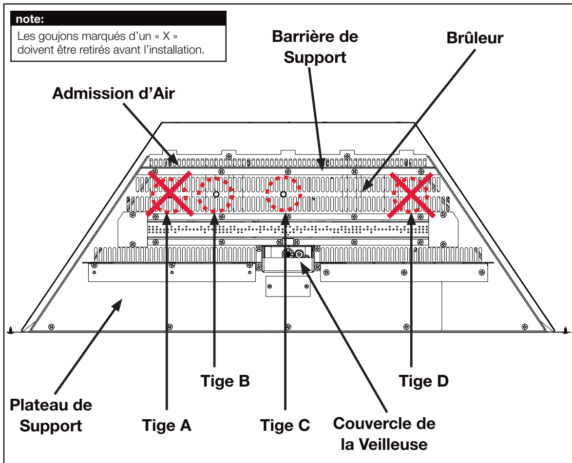
Vue d'Ensemble de Brûleur
