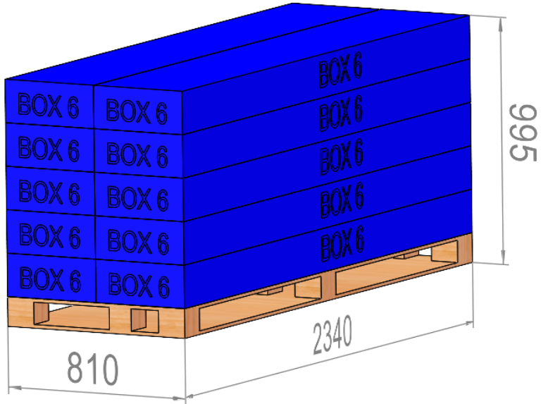
10 boxes per pallet 2 Pallets
