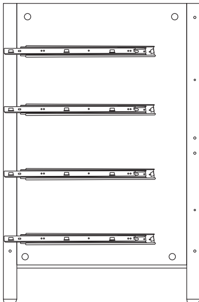
F-3. Left Side Panel F-3. Panneau latéral gauche
