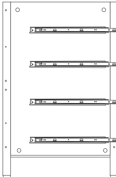
F-4. Right Side Panel F-4. Panneau latéral droit
