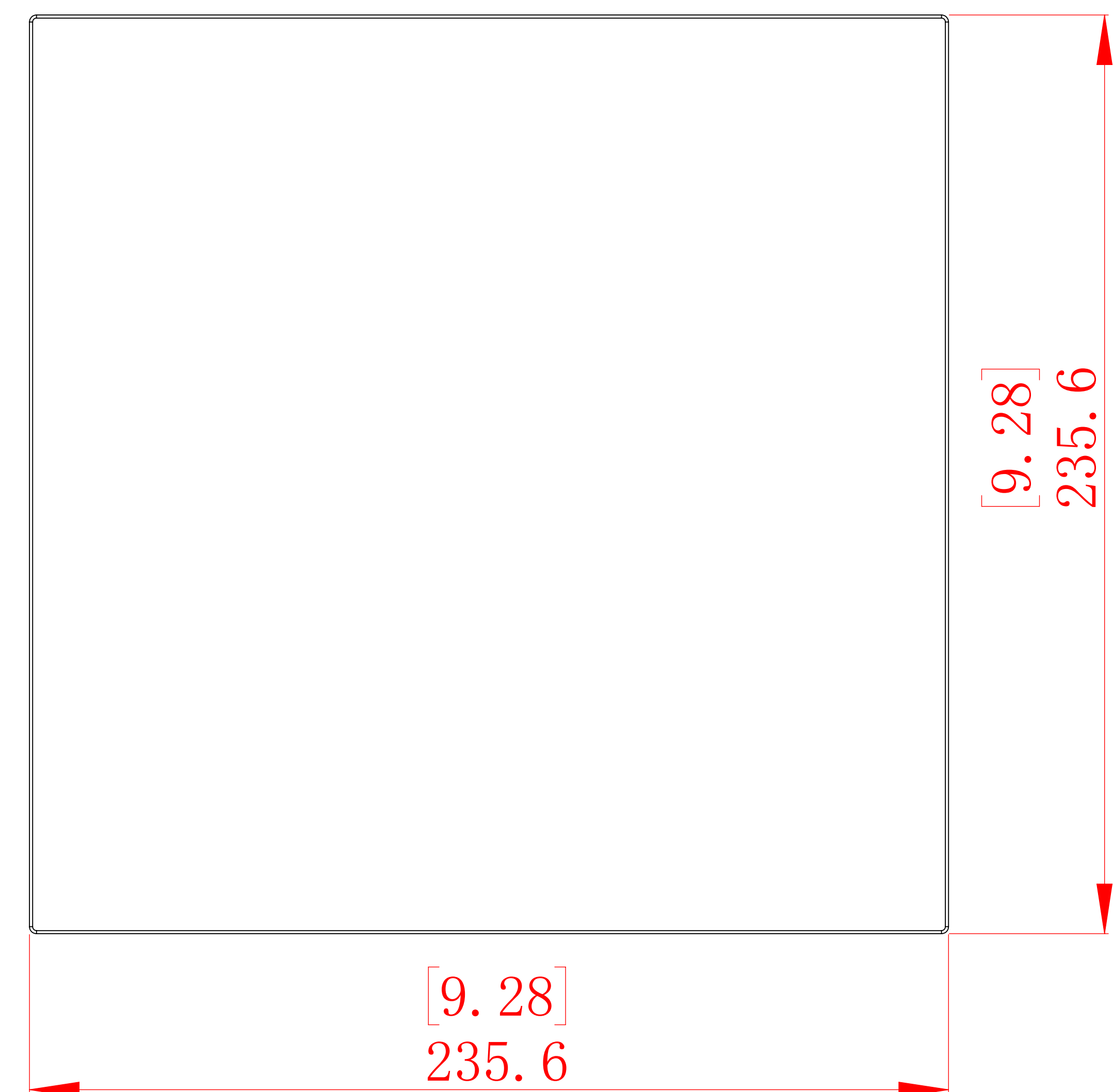
TRIMLESS GRILLE
