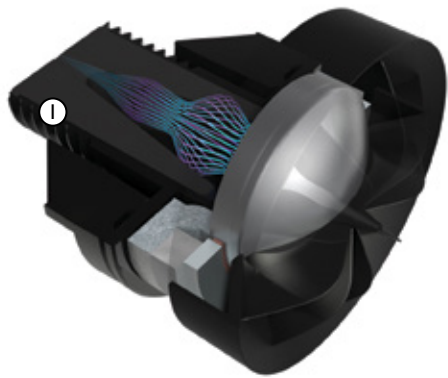
Hochtöner-Aufbau
