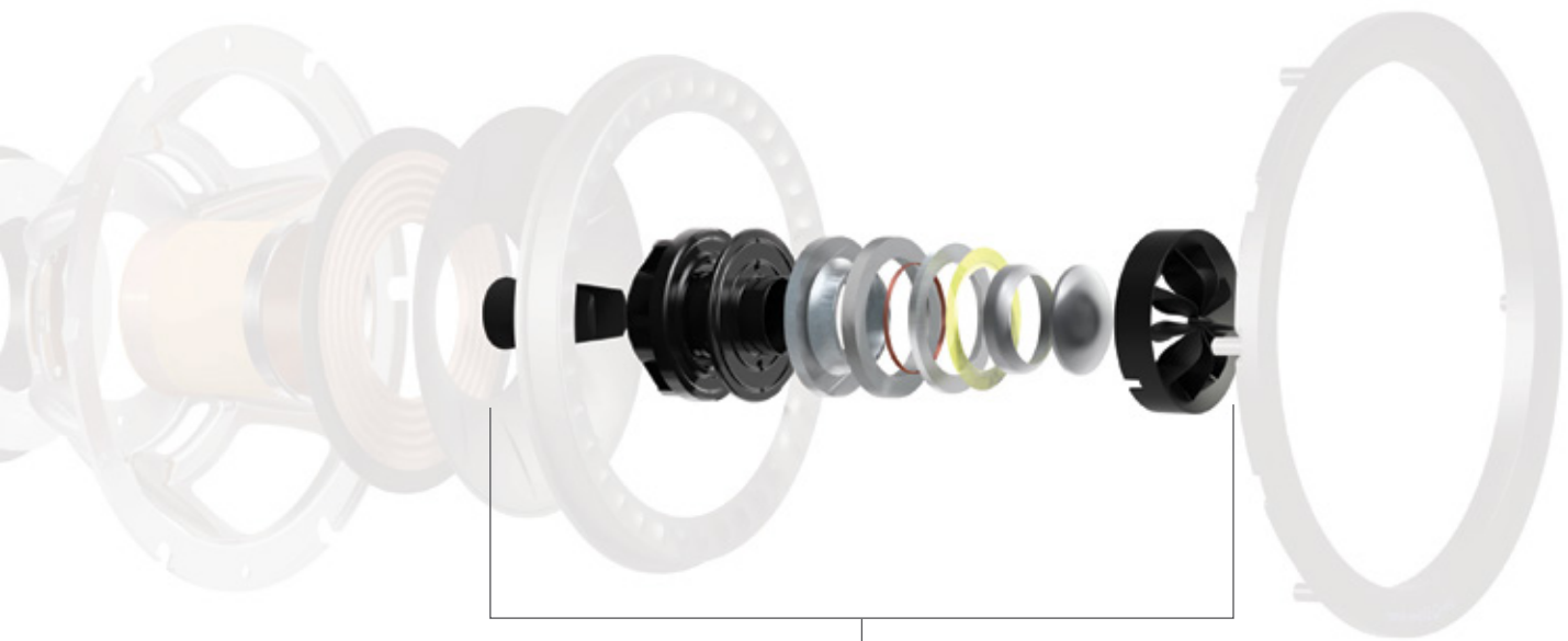
Hochtöner-Aufbau
