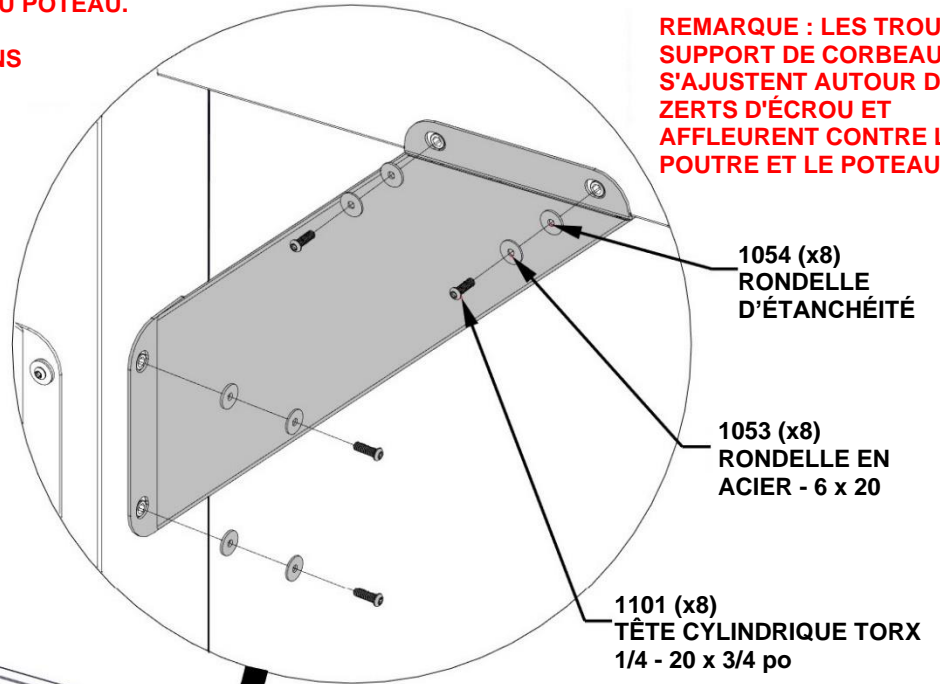
D05 CORBEAU - A4M01831 (x1) 2 3/4 po x 5 7/8 po x 24 13/16 po (70x149x631)
