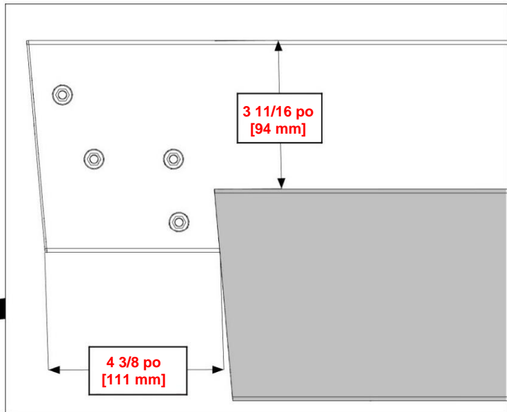
B08 (x1) POUTRE LATÉRALE
