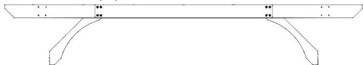
ASSEMBLAGE DE SOLIVES EXTÉRIEURES (x2) - À PARTIR DE L'ÉTAPE 6
