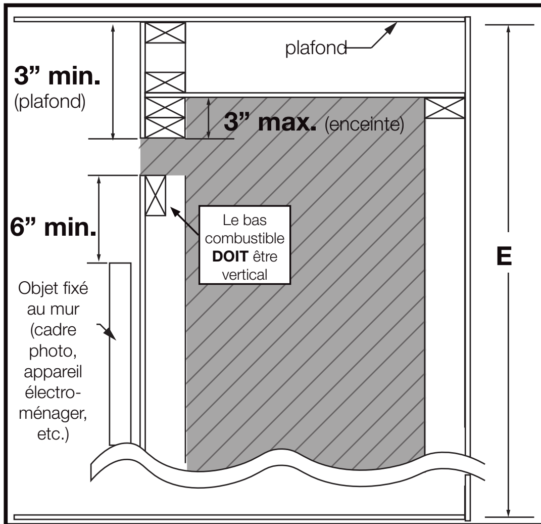
VUE LATÉRALE
