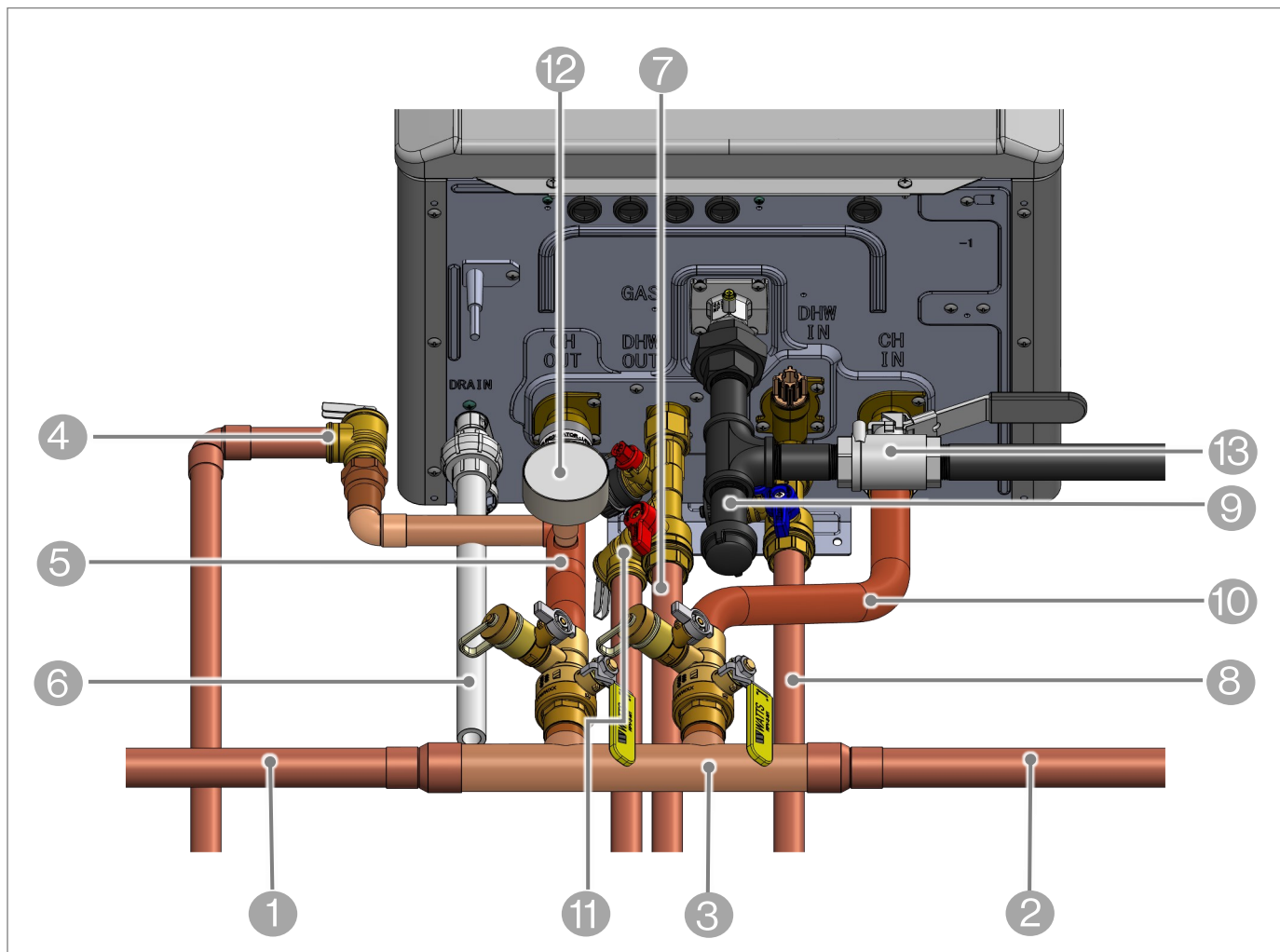
Figure 3: Tuyauterie vue de dessous
