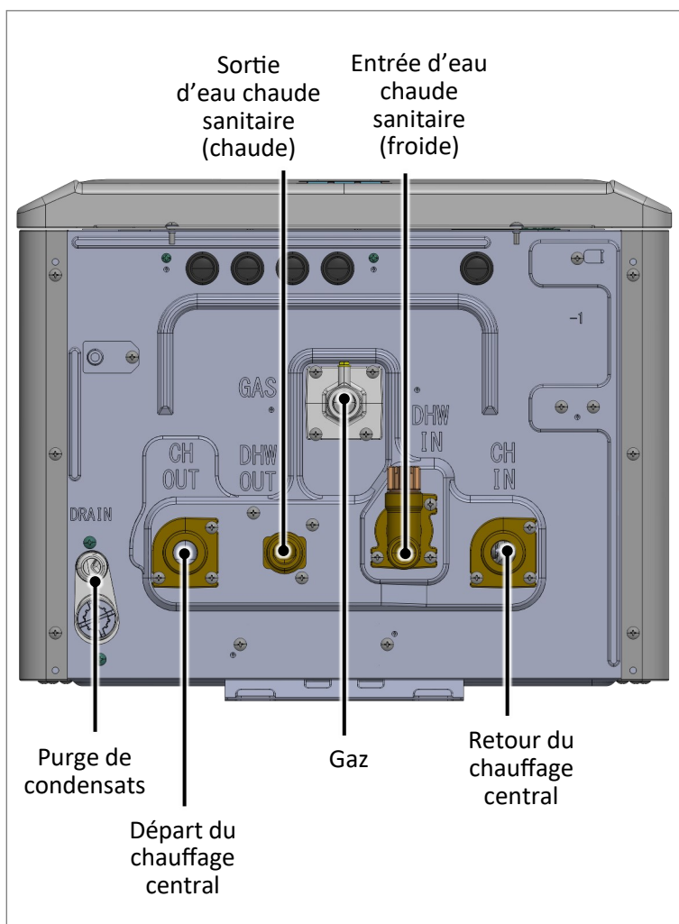
Figure 2: Vue du dessous
